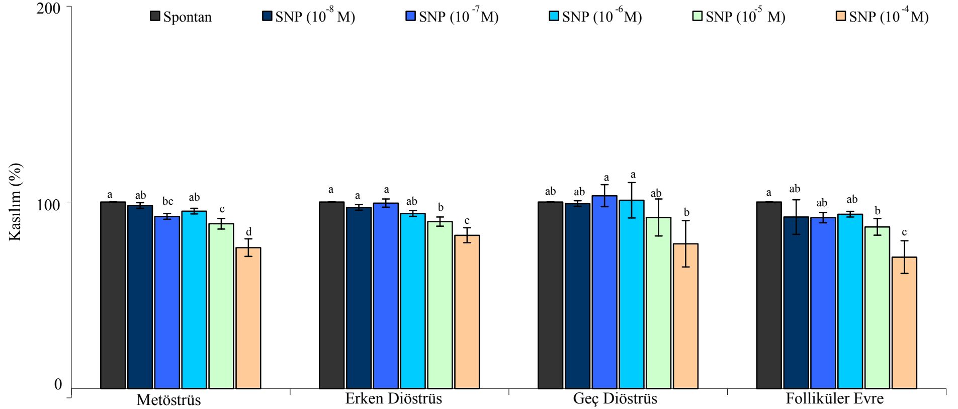
Şekil 3.6: Graplarda istmusun sirküler düz kası üzerine çeşitli konsantrasyonlardaki SNP ( 10^{-8} M, 10^{-7} M, 10^{-6} M, 10^{-5} M, 10^{-4} M) varlığında oluşan yüzde (%) kasılım değerleri. Her bir grupta farklı harfleri taşıyan değerler arasında istatistik olarak fark bulunmuştur ( p < 0.001 ).
