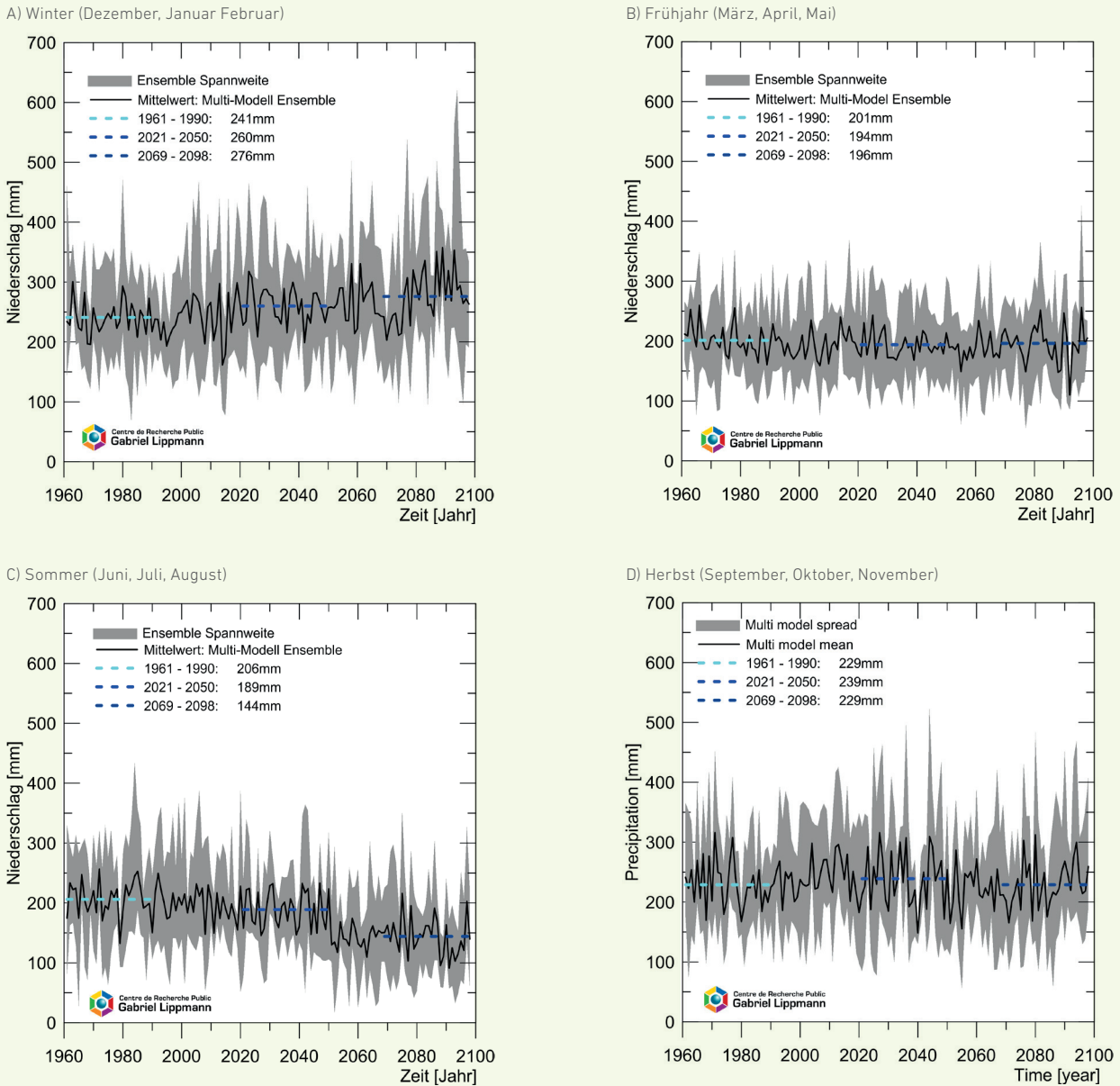
Abb. 2.7 Mittelwerte des Multi-Model Ensembles zu Lufttemperatur und Niederschlag 21
