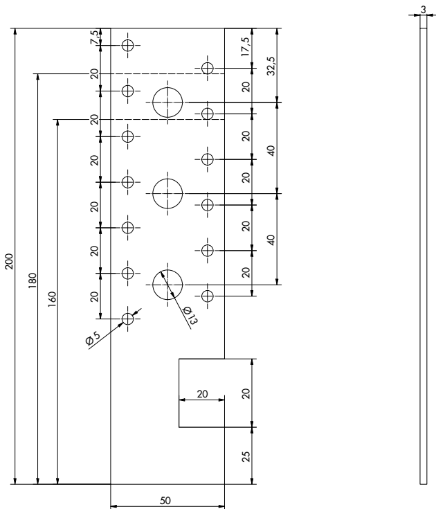
Frontalansicht
