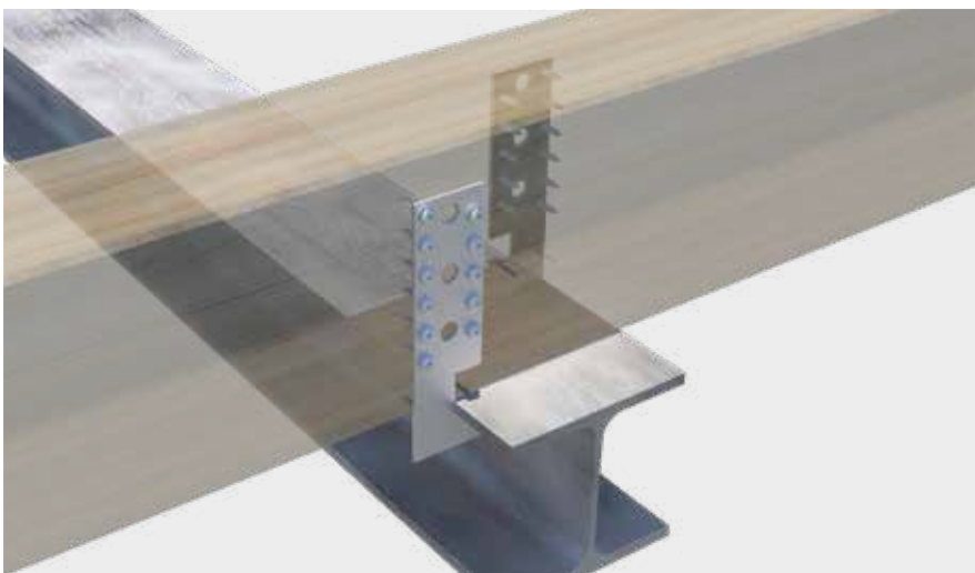
T-Träger Anker in Verbindung mit einem T-Träger.
