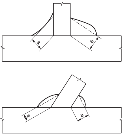
Bild 4.3. Kehlnahtdicke
