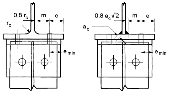
c) Flanschswinkel
