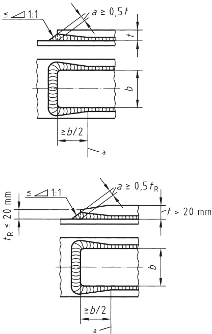
Bild NA.4. Verbinden zusätzlicher Gurtplatten
