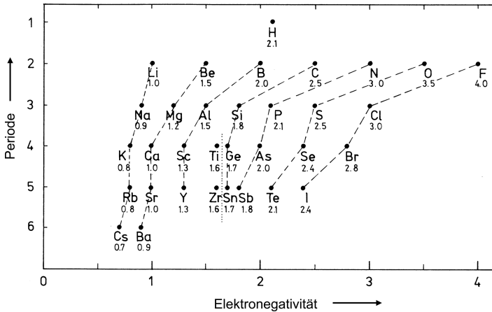
Abb. 1.8 Die Elektronegativitätsskala.
