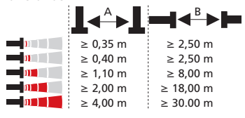
Abb. 1: Montageabstände, unterhalb derer Synchronisation/Multiplex genutzt werden sollte
