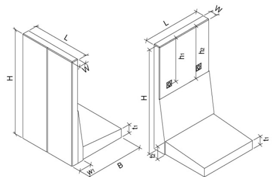
Bild 6: COMOFORTE® Winkelplatte Typ 2
