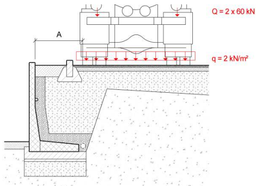
Bild 13: Lastfall C4
