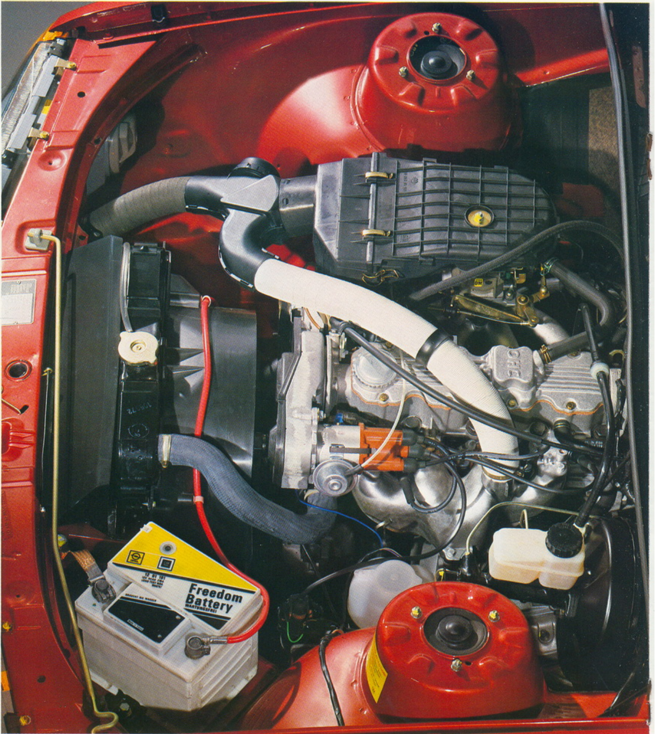
1.8 S-OHC-Motor
