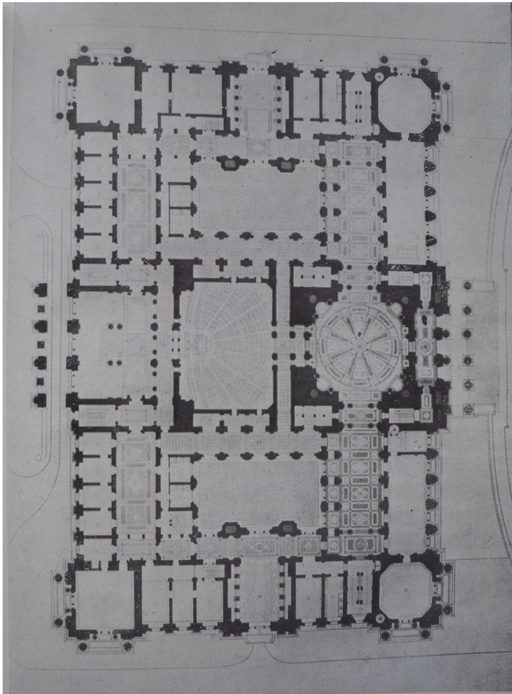
Das Hauptgeschoss des Reichstagsgebäudes im Grundriss
