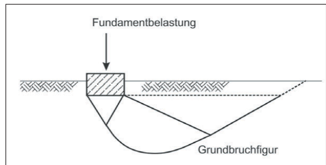
Abb. 6: Beispiel für GZ 1B: Nachweis der Sicherheit gegen Grundbruch
