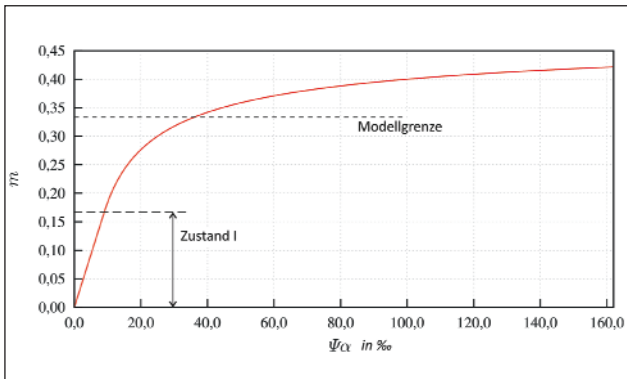
Abb. 12: Beziehung zwischen (bezogenem) Rückstellmoment und Verdrehung
