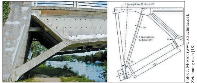
Abb. 2: Auflagerbereich der Marne-Brücken mit Betongelenk nach Freyssinet
