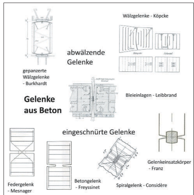
Abb. 3: Klassifikation der Gelenke aus Beton
