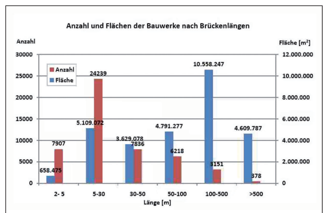
Abb. 10: Bauwerksbestand nach Brückenlängen
