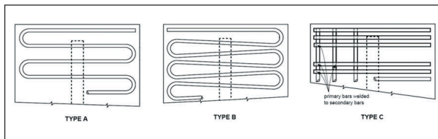
Abb. 8: Mögliche Bewehrungsformen des britischen Modells (aus [10])
