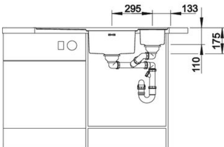
Frontansicht
