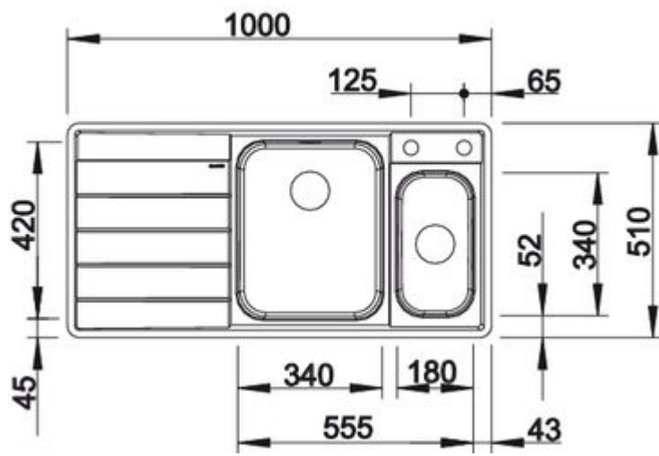
Draufsicht
