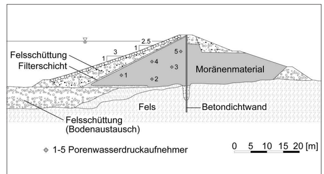
Bild 7: Querschnitt Glen Shira Dammbauwerk nach Paton & Semple (1961)
