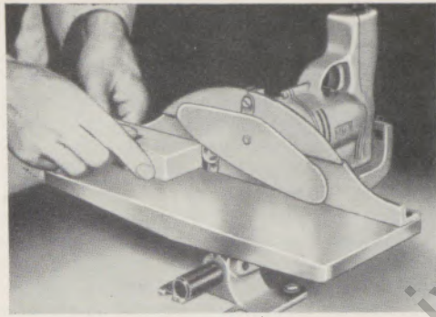
Hobelmaschine
