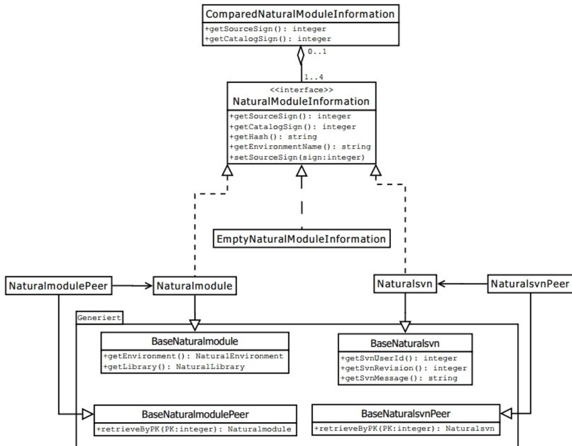
Abbildung 11: Klassendiagramm
