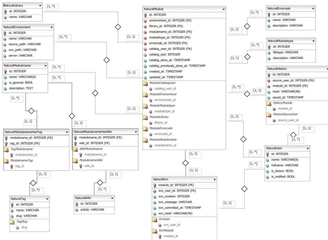
Abbildung 3: Tabellenmodell
