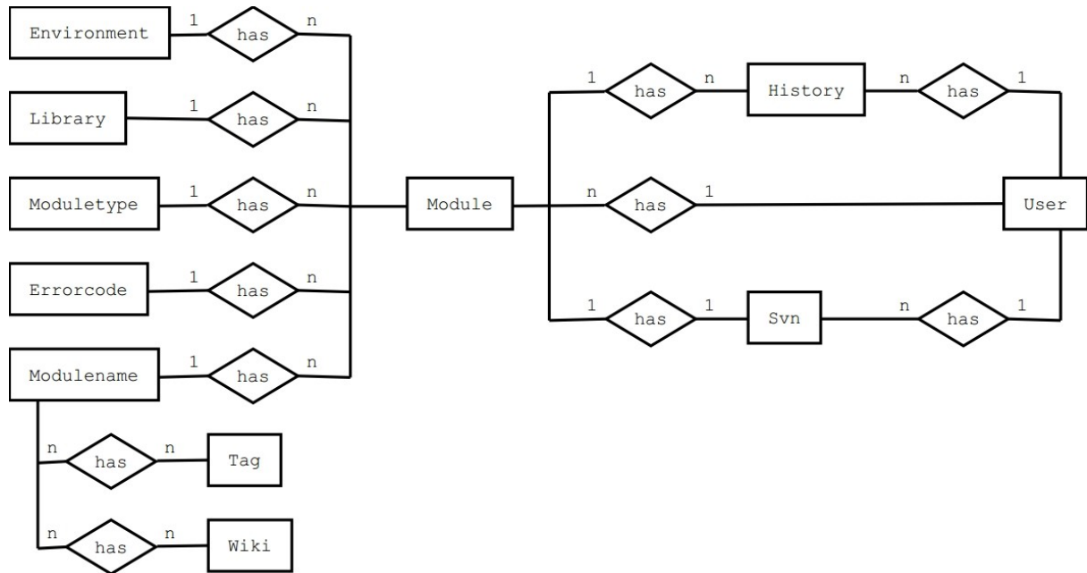
Abbildung 2: Entity-Relationship-Model
