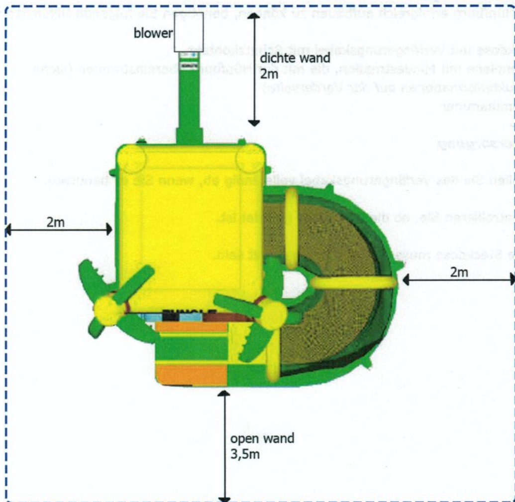
Abbildung 2 Mindestens erforderlicher Freiraum um die Hüpfburg herum (Beispiel allgemeine Hüpfburg).
