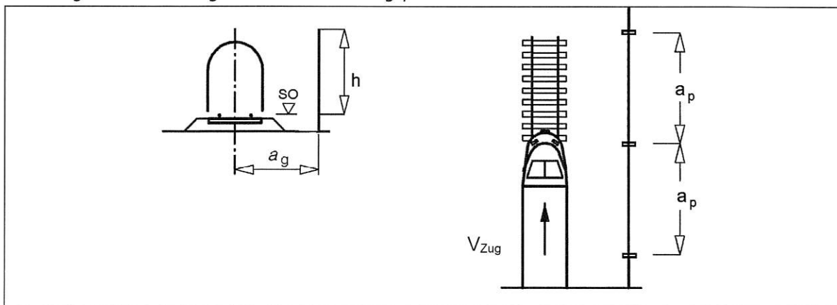
Abbildung 1: Bemessungsrelevante Trassierungsparameter
