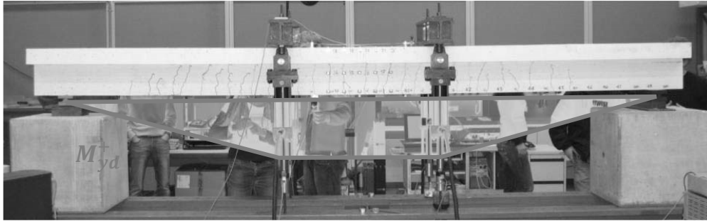
Angestrebte Bruchart (duktil): Betonbruch während Stahlfließens:
