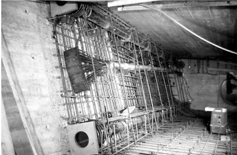
Reussbrücke Wassen – Reparaturarbeiten
