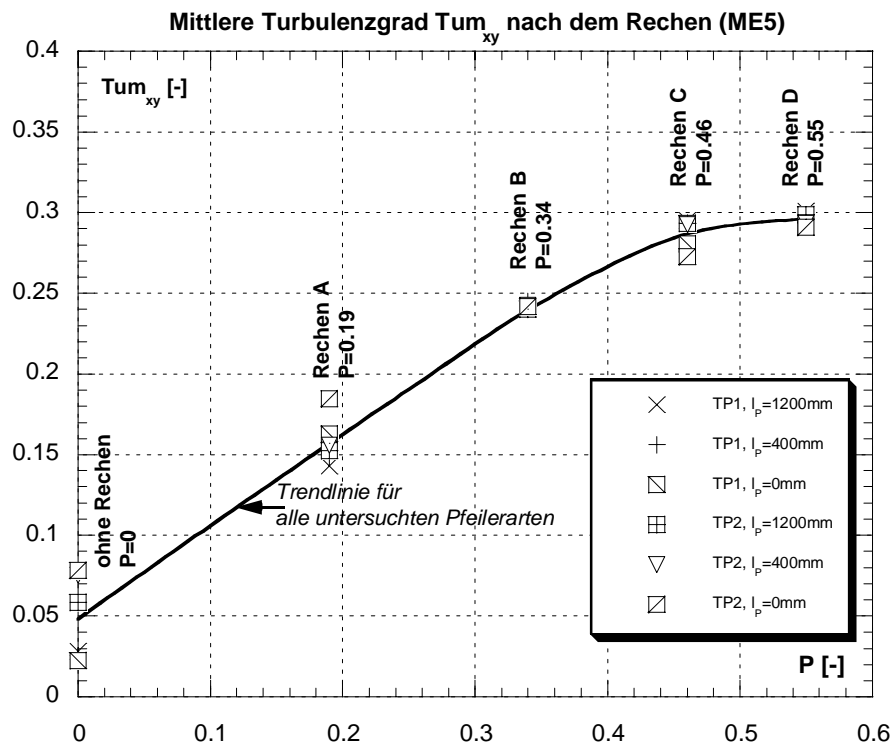
Abb. 4.37: Mittlerer Turbulenzgrad Tum_{xy} für die untersuchten Trennpfeilerformen unmittelbar nach dem Rechen (ME5) in Abhängigkeit des Verbaungsgrades P .
