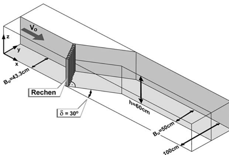
Abb. 4.8: Modellierung der Schräganströmung für \delta = 30^\circ .
