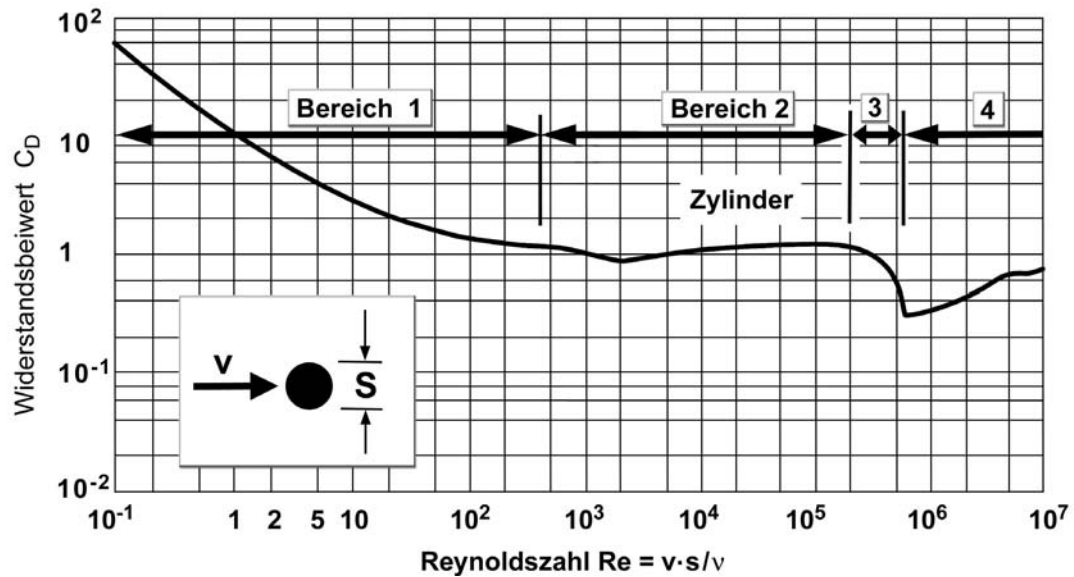
Abb. 3.2: Widerstandsbeiwert eines Kreiszyinders in Abhängigkeit von der Reynoldszahl nach Blevins (1984).
