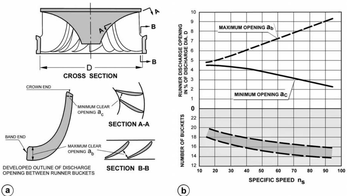
Abb. 2.17: a) Lage der kleinsten und grössten freien Durchflussöffnung bei einer Francisturbine. b) Erfahrungswerte für eine erste Näherungsberechnung der kleinsten und grössten freien Durchflussöffnung für eine Francisturbine nach Zowski (1960).
