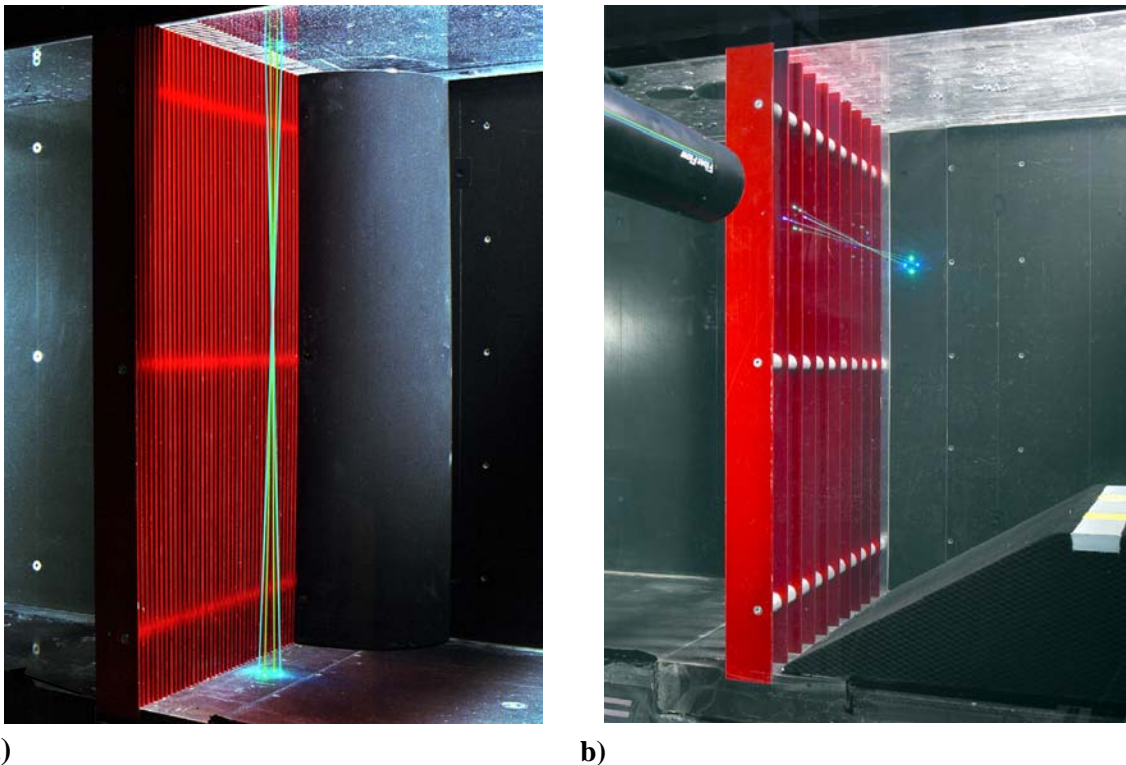
Abb. 4.32: Geschwindigkeitsmessung mittels der LDA-Anlage a) in der horizontalen x-y-Ebene für einen abgerundeten Trennpfeiler des Typ TP1 mit l_p=0\text{mm} und Rechen D b) in der vertikalen x-z-Ebene mit eingebauter Sohlenform des Typ ES3 und Rechen B.
