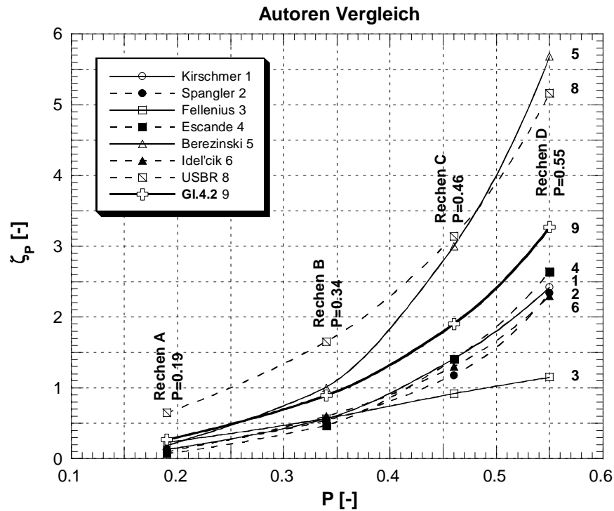
Abb. 4.5: Vergleichende Darstellung der berechneten Verlustbeiwerte \zeta_p in Abhängigkeit des Verbaugungsgrades P nach verschiedenen Autoren für die einzelnen Rechen.
