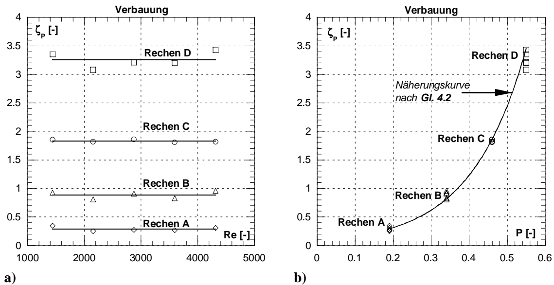
Abb. 4.4: a) Abhängigkeit des Verlustbeiwertes \zeta_p von der Reynolds-Zahl Re (Geschwindigkeit) für die Rechen A bis D. b) Darstellung des Verlustbeiwertes \zeta_p in Abhängigkeit des Verbaugrades P mit der ermittelten Näherungskurve nach Gl. 4.2 für die Rechen A bis D nach Gl. 4.2.
