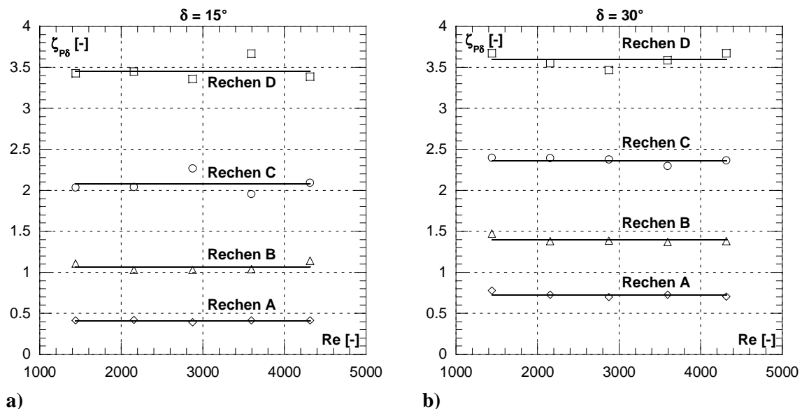
Abb. 4.10: Abhängigkeit des Verlustbeiwertes \zeta_{P\delta} von der Reynolds-Zahl Re . a) für einen Schräganströmwinkel \delta=15^\circ , b) für einen Schräganströmwinkel \delta=30^\circ .
