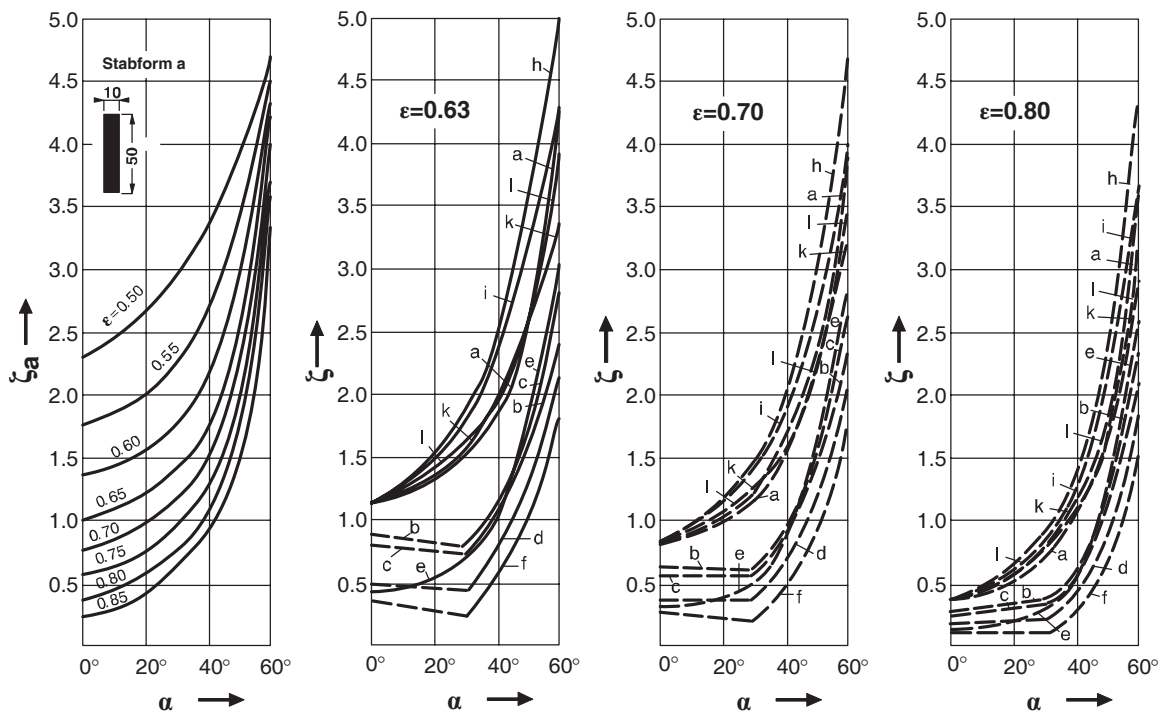
Abb. 2.30: Diagramme zur Bestimmung des Verlustkoeffizienten \zeta bzw. \zeta_a in Abhängigkeit der untersuchten Stabformen a bis l, des ‘Durchflussverhältnisses’ \epsilon und dem Winkel der mittleren Schräganströmung \alpha ( Spangler , 1928). Das erste Diagramm für \zeta_a (links) gilt nur für die Stabform a.
