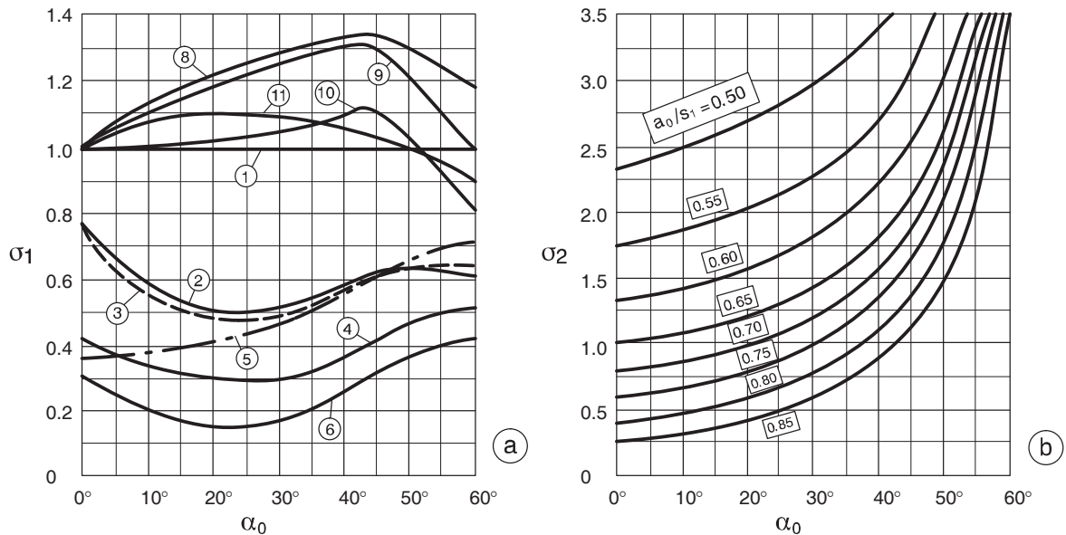
Abb. 2.35: a) Verlustbeiwert \sigma_1 in Funktion des horizontalen Anströmwinkels \alpha_0 und der Stabform. b) Verlustbeiwert \sigma_2 in Funktion des horizontalen Anströmwinkels \alpha_0 und des Verhältnisses a_0/s_1 (Idel'cik, 1979).
