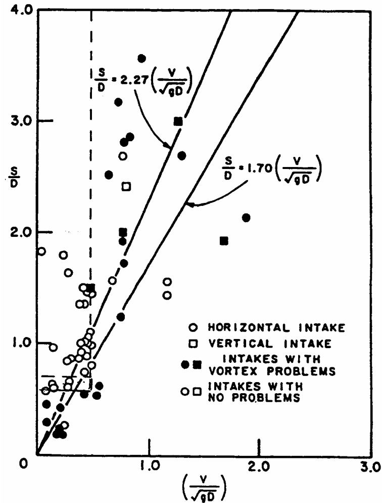
Abb. 2.27: Bedingung zur Vermeidung von Einlaufwirbeln nach Gulliver et al. (1983).
