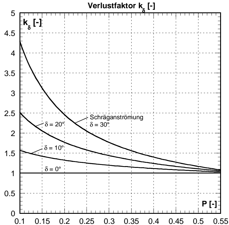
Abb. 5.4: Abhängigkeit des Verlustfaktors k_\delta vom Verbauungsgrad P und dem Winkel der Schräganströmung \delta .
