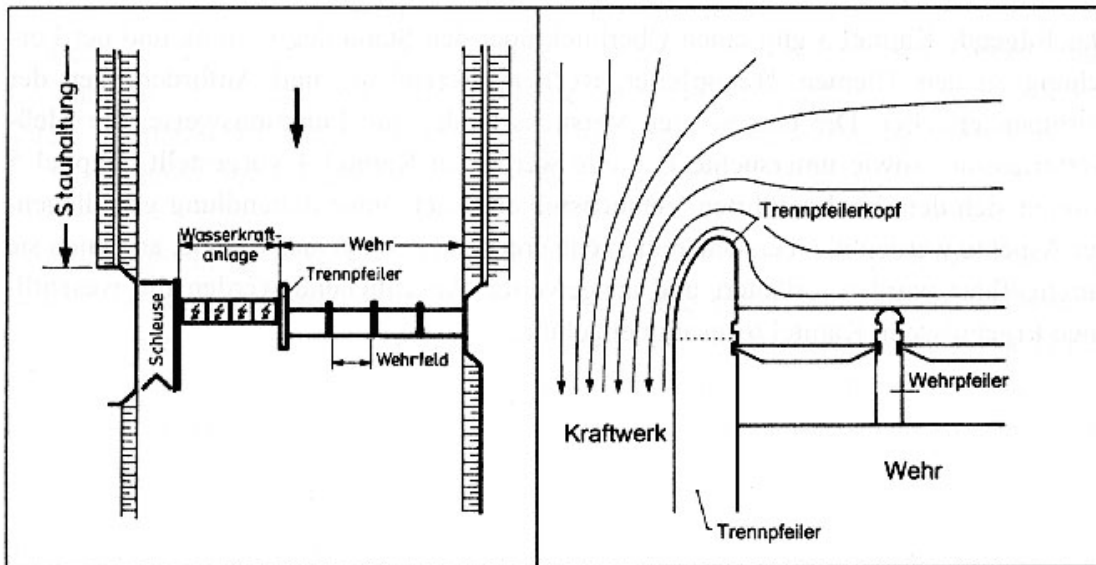
Abb. 4.27: Anordnung des Trennpfeilers bei einem Blockkraftwerk.
