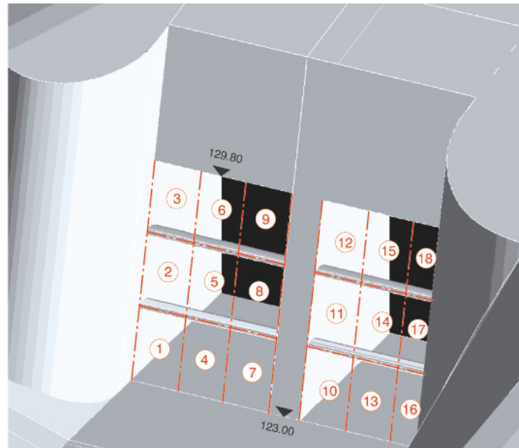
Abb. 5.11: Mögliche Aufteilung eines Rechenfeldes in Teilfelder.
