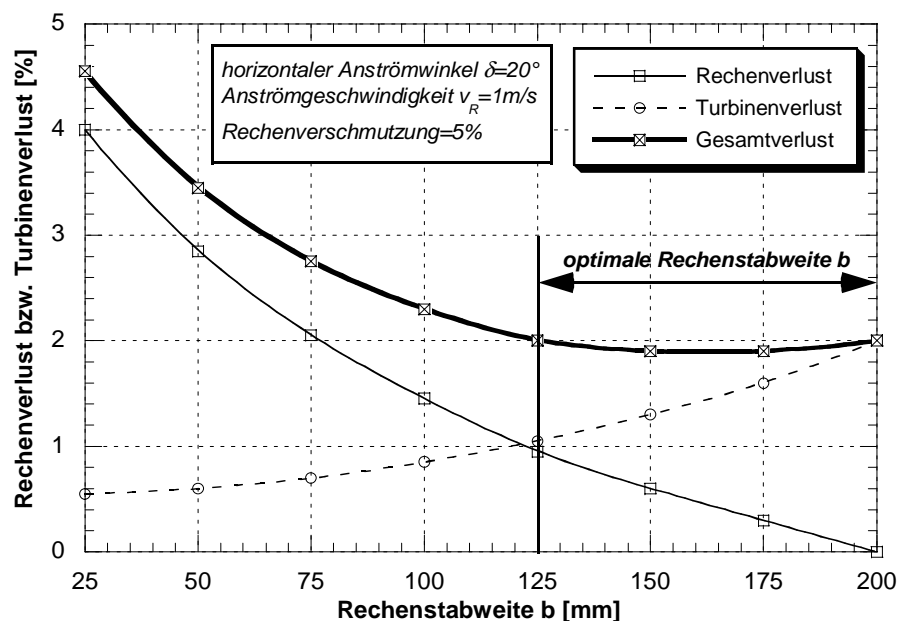
Abb. 2.23: Einfluss der Schräganströmung auf Rechenverlust und Turbinenwirkungsgrad bei einem horizontalen Anströmwinkel d=20^\circ , einer Anströmgeschwindigkeit v_R = 1 \text{ m/s} und einer Rechenverschmutzung von 5% der noch freien Durchgangsfläche, in Abhängigkeit der lichten Rechenstabweite b ( Sulzer-Hydro , 1995)
