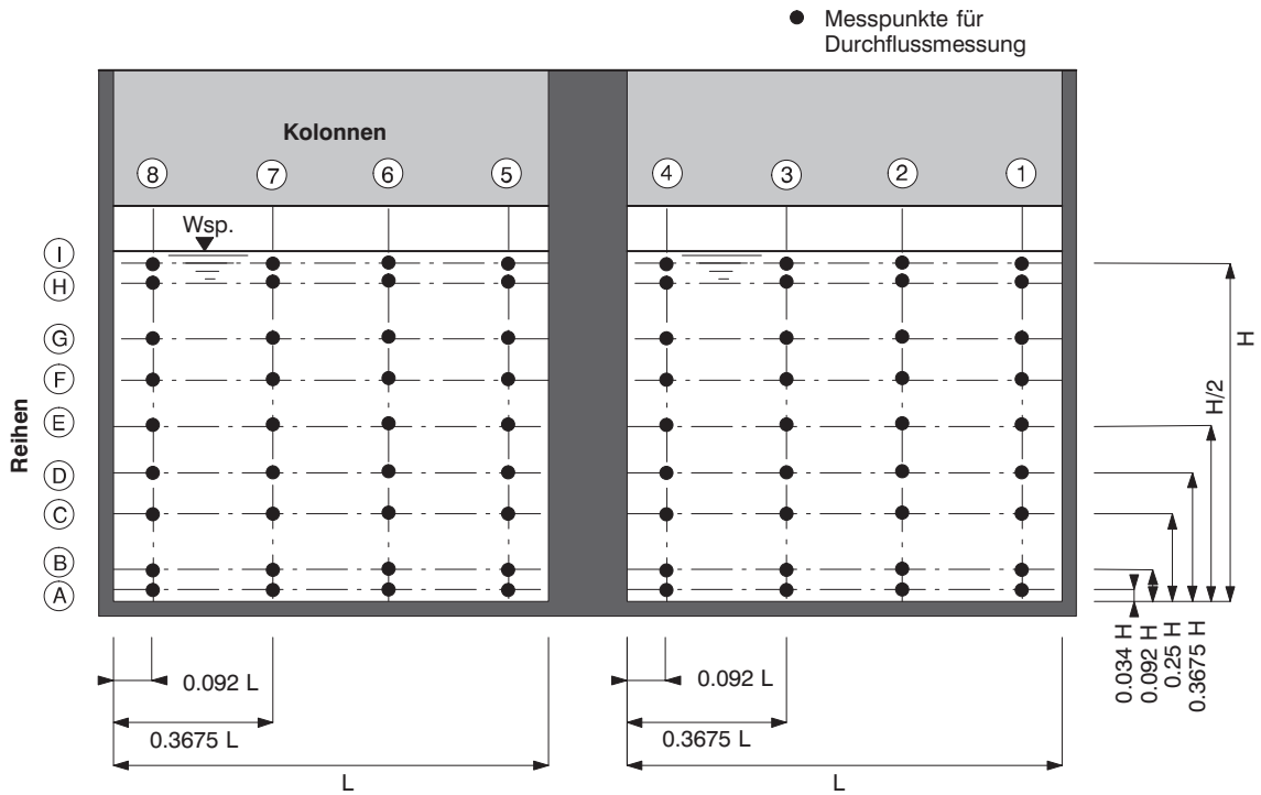
Abb. C.3: Allgemeiner Messraster nach ISO 3354 (1975).
