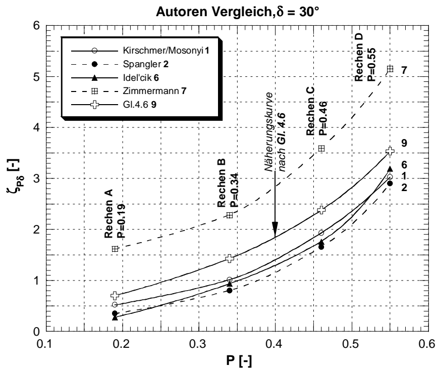
Abb. 4.14: Vergleichende Darstellung der am Modell gewonnenen Ergebnisse (Gl. 4.6) mit berechneten Verlustbeiwerten \zeta_{P\delta} für \delta=30^\circ in Abhängigkeit des Verbauungsgrades P nach verschiedenen Autoren.
