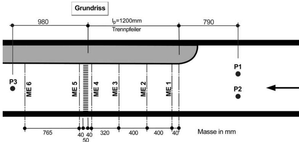
Abb. 4.33: Anordnung der Messebenen im Grundriss für l_p = 1200\text{mm} .
