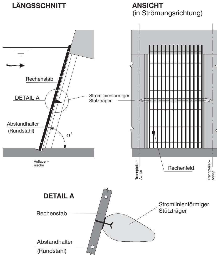
Abb. 2.3: Schema der Rechenkonstruktion mit waagrechtter Abstützung der Rechentafeln.
