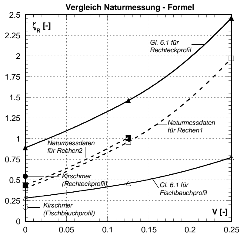
Abb. 6.10: Vergleich der Verlustbeiwerte aus der Naturmessung und Berechnungen nach Kirschmer und Gl. 6.1 in Abhängigkeit der Verlegung V . Die durchgezogenen Linien entsprechen Berechnungen und die gestrichelten denen der Naturmessung.
