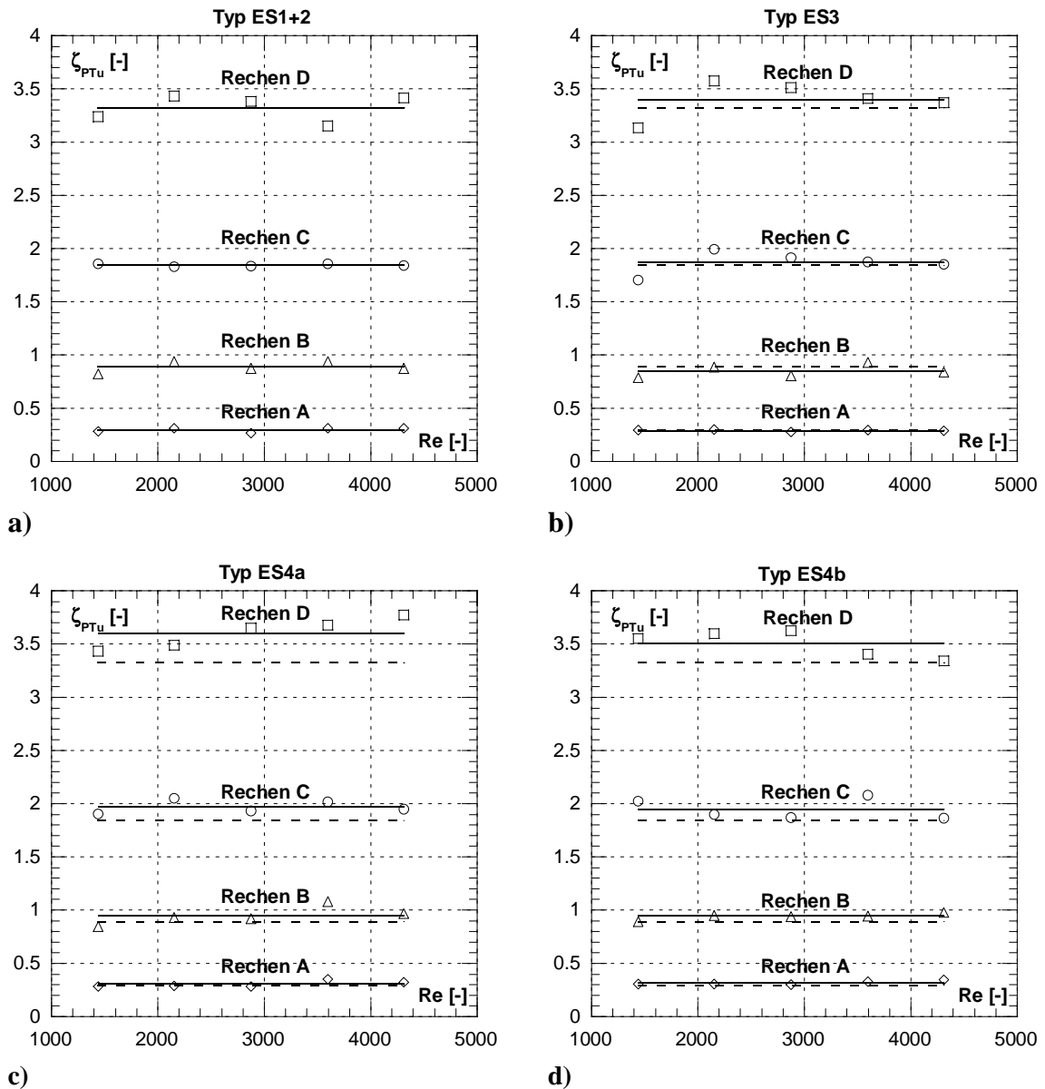
Abb. 4.40: Verlustbeiwert \zeta_{PTu} infolge Verbauung P und Turbulenz Tu in Abhängigkeit der Rechenstab-Reynoldszahl Re für die untersuchten Einlaufsohlenformen. Gestrichelte Linie entspricht Verlustbeiwert \zeta_P infolge Verbauung P allein, durchgezogene Linie entspricht Verlustbeiwert \zeta_{PTu} infolge Verbauung P und Turbulenz Tu.
