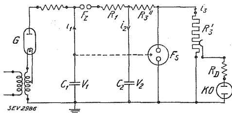
Fig. 13. Schema zur Untersuchung der Funkenstrecke F_s bei flachen Wellen (Überschläge von F_s in der Spannungsfrent).
