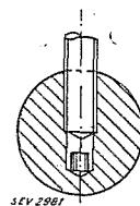
Fig. 2. Radiumionisierte Kugelelektrode.
