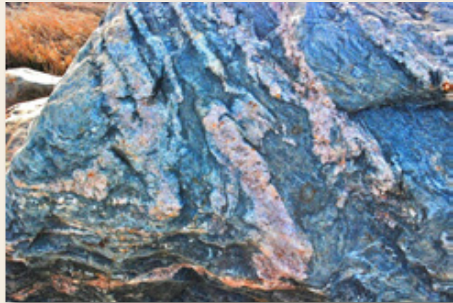
Migmatit
