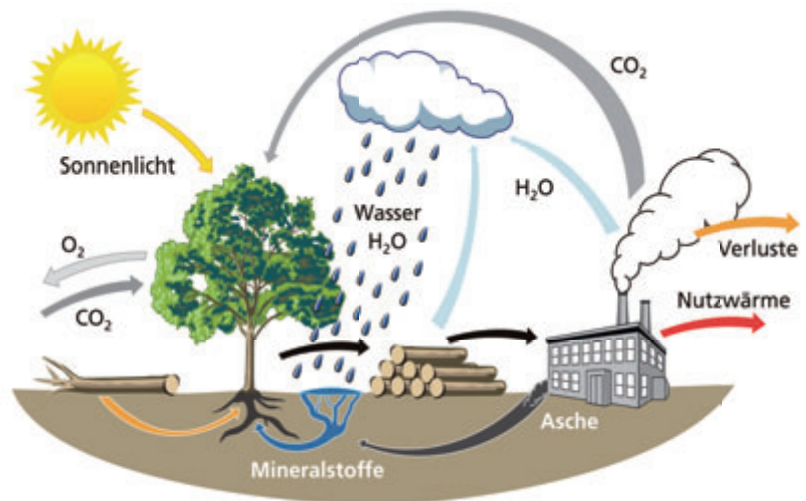
Abb. 1.4: Kohlenstoffkreislauf
