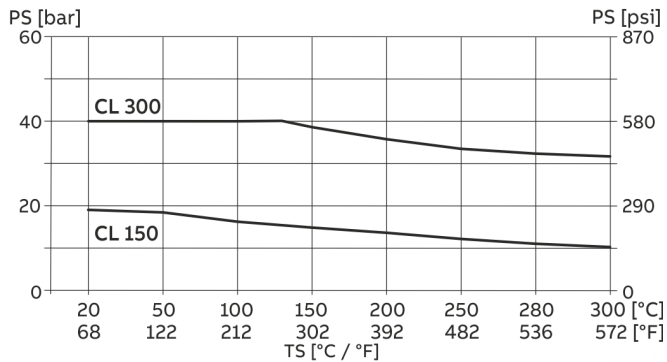
Abbildung 17: Prozessanschluss ASME-Flansch
