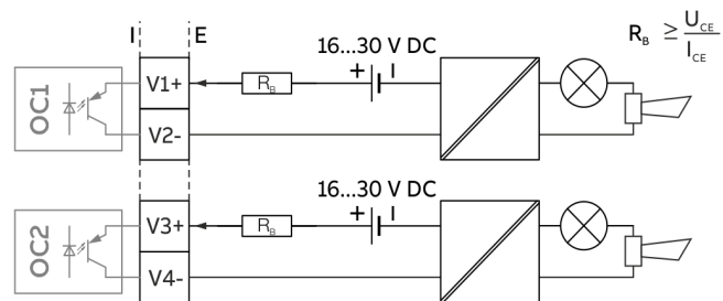
Abbildung 60: Einsteckkarte als Binärausgang (I = Intern, E = Extern, R_B = Bürde)
