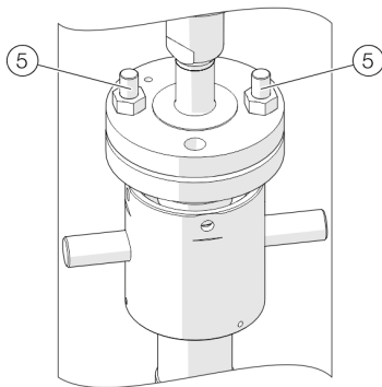
Abbildung 35: Flanschschrauben entfernen
