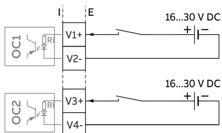
Abbildung 61: Einsteckkarte als Digitaleingang (I = Intern, E = Extern)
