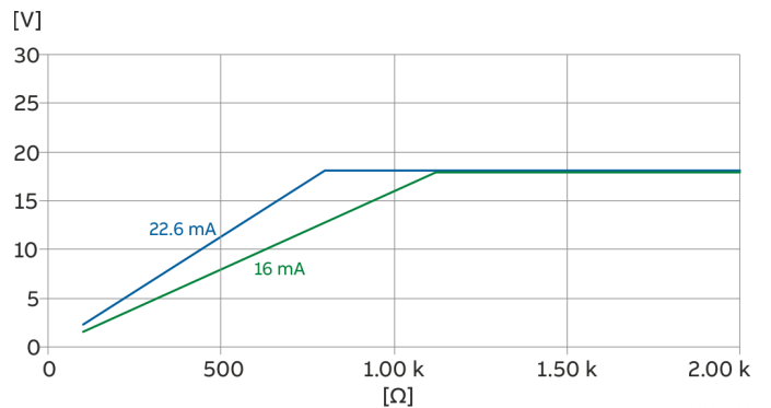
Abbildung 55: Ausgangsspannung abhängig vom Bürdenwiderstand
