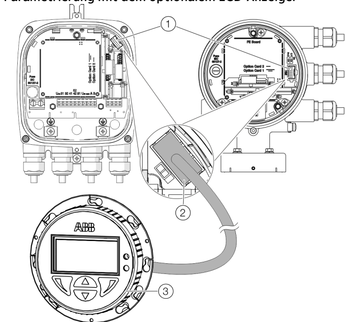
Abbildung 79: Anschluss an der lokalen Bedienschnittstelle
