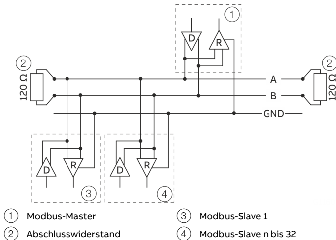
Abbildung 73: Kommunikation mit Modbus-Protokoll
