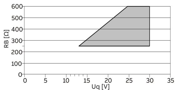
Abbildung 52: (I = Intern, E = Extern, R_B = Bürde)
