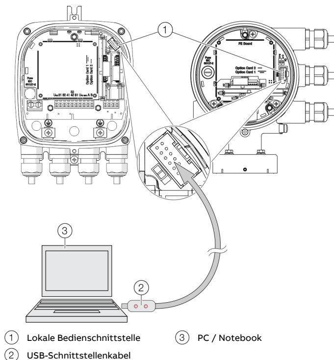
Abbildung 79: Anschluss an der lokalen Bedienschnittstelle
