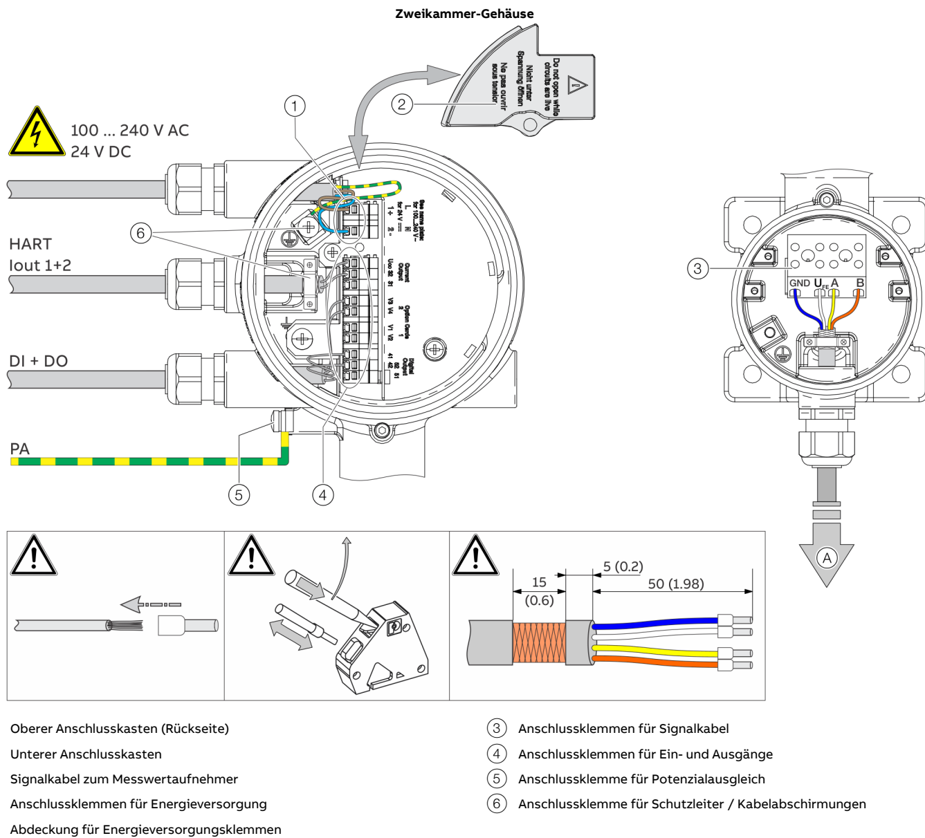
Abbildung 70: Elektrischer Anschluss Messumformer in getrennter Bauform [Beispiel, Abmessungen in mm (in)]
