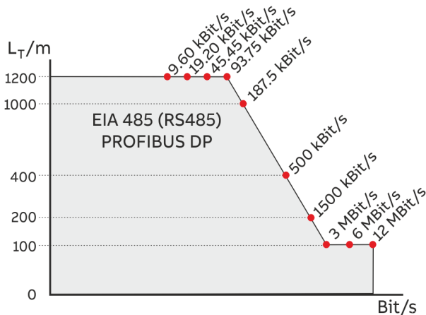
Abbildung 74: Buskabellänge in Abhängigkeit zur Übertragungsrate
