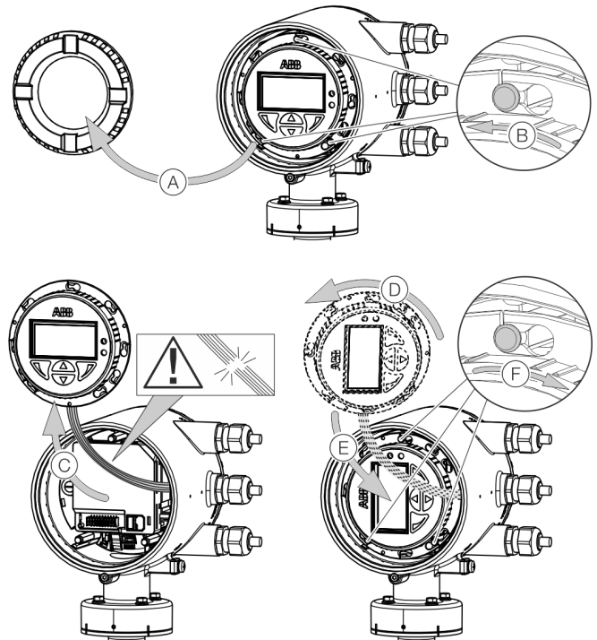
Abbildung 46: LCD-Anzeiger drehen
