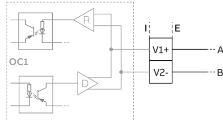
Abbildung 57: Einsteckkarte als Modbus- / PROFIBUS DP-Schnittstelle (I = Intern, E = Extern)
