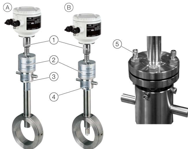
Abbildung 29: Messwertaufnehmer-Verbindung an der Wechselvorrichtung
