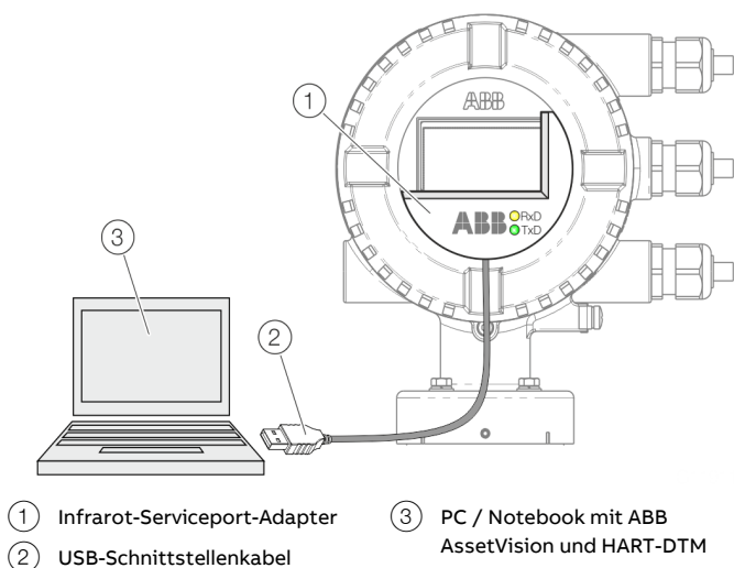
Abbildung 80: Infrarot-Serviceport-Adapter am Messumformer (Beispiel)
