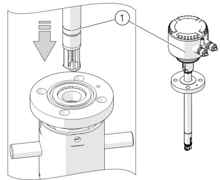
Abbildung 37: Messwertaufnehmer einschieben
