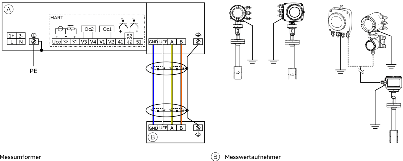
Abbildung 51: Anschlussplan
