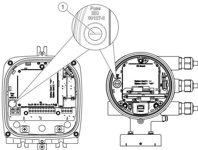
Abbildung 86: Position Sicherungshalter
