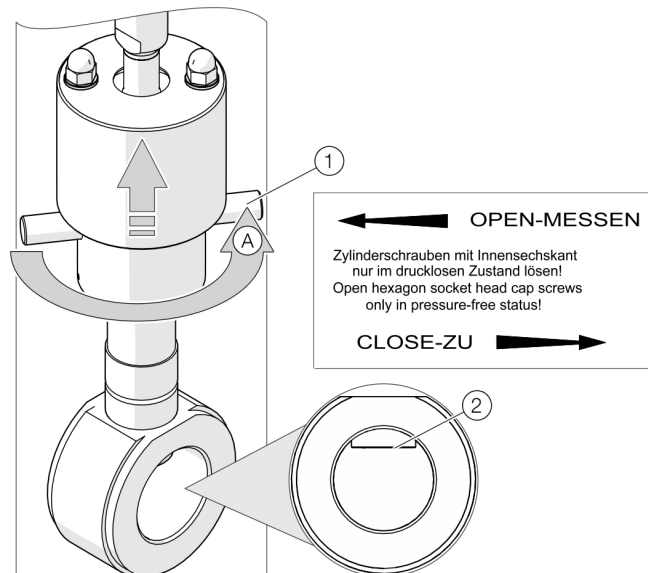
Abbildung 32: Integrierte Wechsellvorrichtung in Ausbauposition bringen
