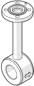
FMT091 – Zwischenflanschführung
