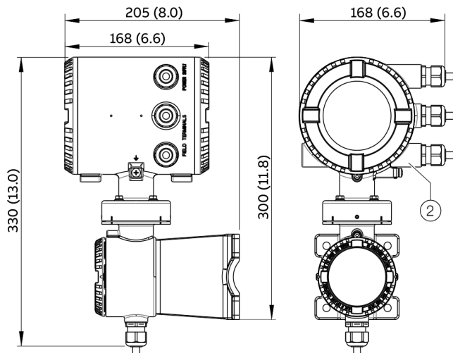
Abbildung 42: Montageabmessungen Einkammer-Gehäuse
