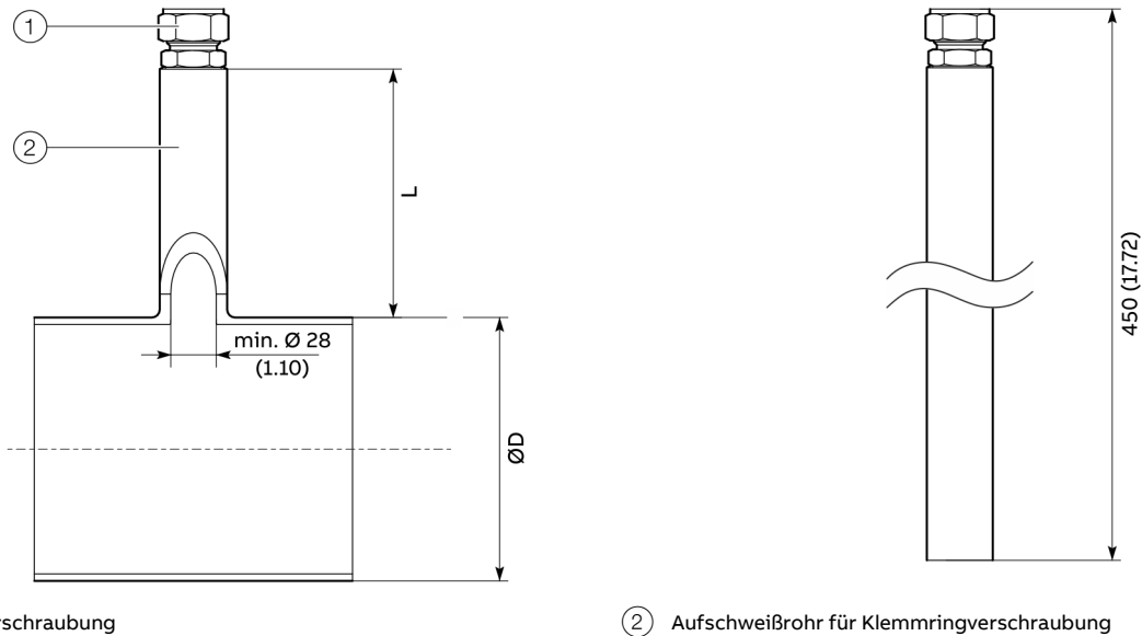
Abbildung 23: Aufschweißadapter mit Klemmringverschraubung
