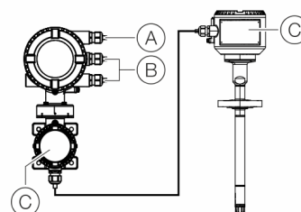
Getrennte Bauform
