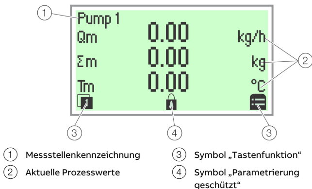
Abbildung 83: Prozessanzeige (Beispiel)
