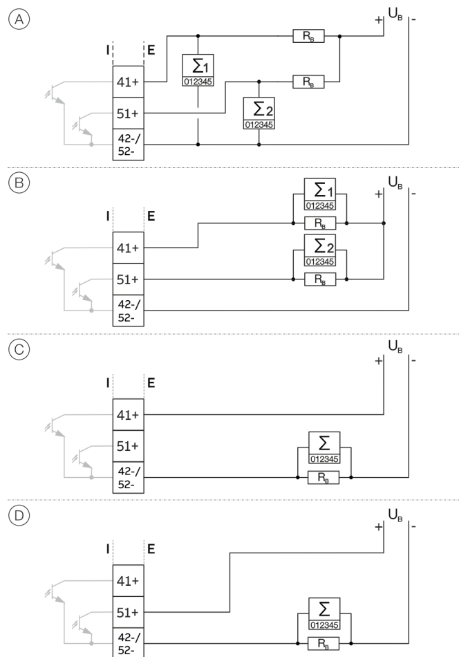
Abbildung 68: Anschlussvarianten Digitalausgang 41 / 42 und 51 / 52
