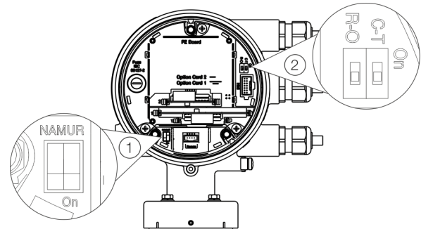
Abbildung 75: Position der DIP-Schalter
