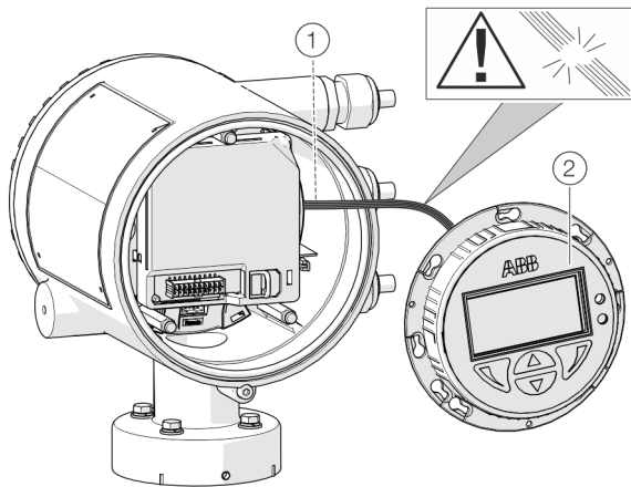
Zweikammergehäuse
