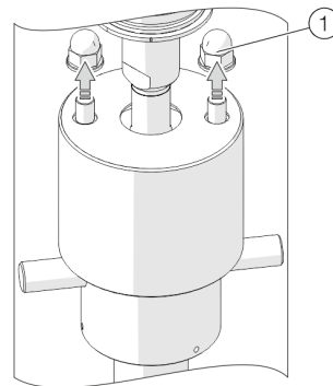
Abbildung 33: Hutmutter der Schutzkappe lösen
