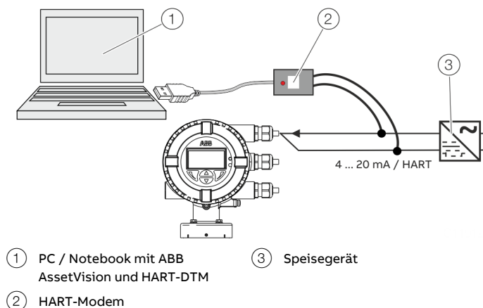
Abbildung 81: HART-Modem am Messumformer (Beispiel)
