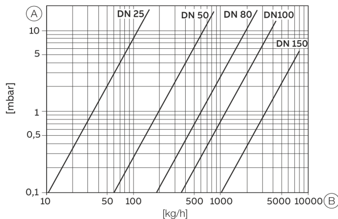
Abbildung 15: Druckverlust in logarithmischer Darstellung
