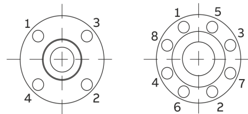
Abbildung 19: Anzugsreihenfolge der Flanschschrauben
