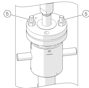
Abbildung 38: Flanschschrauben einschrauben
