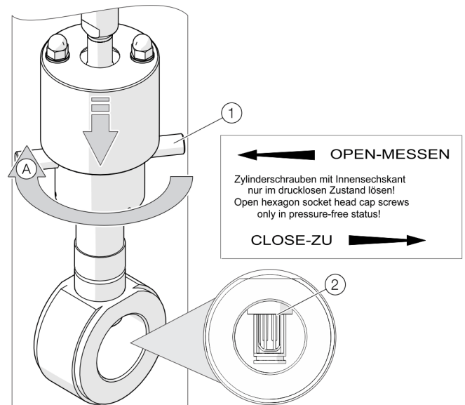
Abbildung 40: Integrierte Wechsellvorrichtung in Messposition bringen
