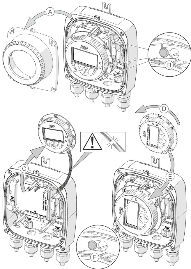
Abbildung 47: LCD-Anzeiger drehen
