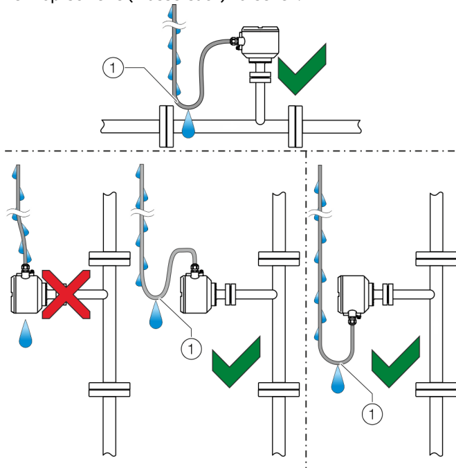
Abbildung 50: Verlegung der Anschlusskabel
