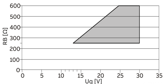
Zulässige Quellenspannung U_q für passive Ausgänge in Abhängigkeit des Bürdenwiderstandes R_B bei I_{max} = 22 \text{ mA} . = Zulässiger Bereich
