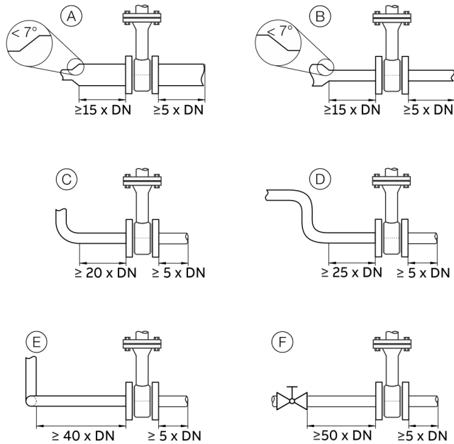
Abbildung 12: Vorlauf- und Nachlaufstrecken
