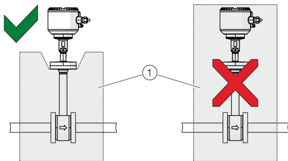
① Isolierung
