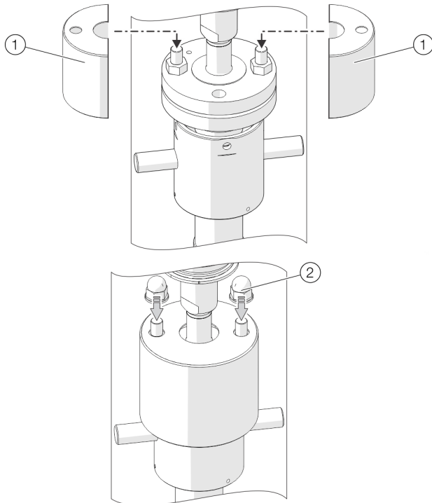
Abbildung 39: Schutzkappen aufsetzen
