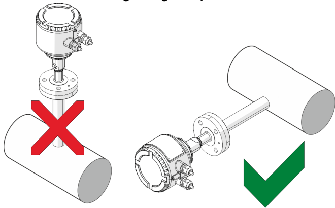
Abbildung 13: Einbaulage bei hohen Umgebungstemperaturen
