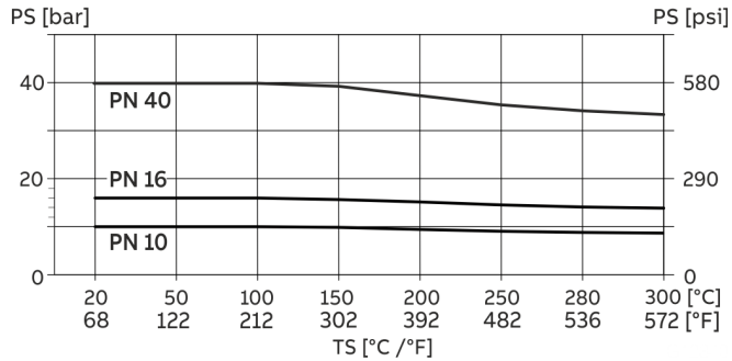
Abbildung 16: Prozessanschluss DIN-Flansch
