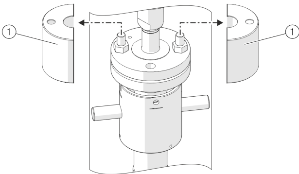
Abbildung 34: Schutzkappen entfernen
