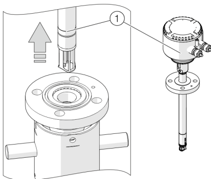
Abbildung 36: Messwertaufnehmer herausziehen
