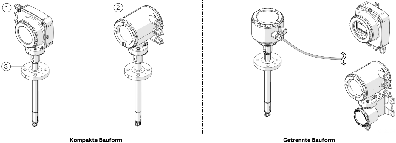
Abbildung 5: Messwertaufnehmer FMT430, FMT450 (Beispiel)
