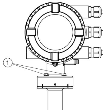
Abbildung 4: Schrauben am Zweikammer-Messumformergehäuse
