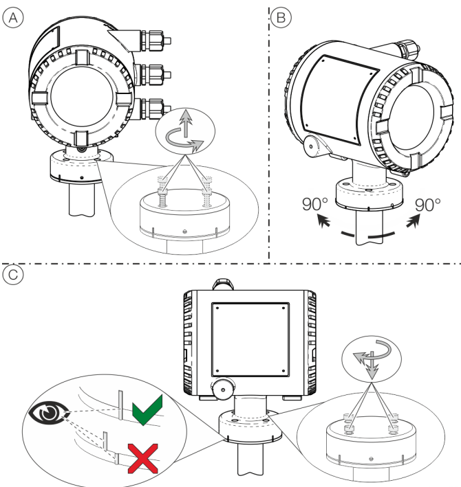
Abbildung 45: Messumformergehäuse drehen
