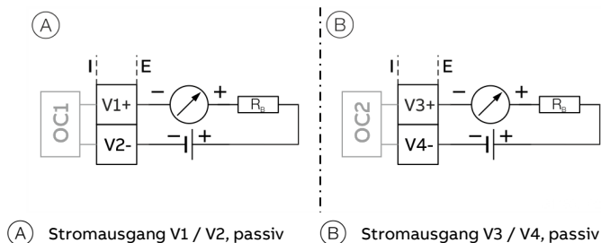
Abbildung 58: (I = Intern, E = Extern, R_B = Bürde)
