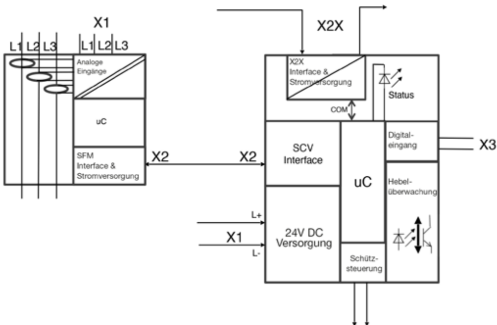
02: Blockschaltbild von SFM1 und SCV. Beide Geräte sind mit einer seriellen Schnittstelle zum Datenaustausch verbunden.
