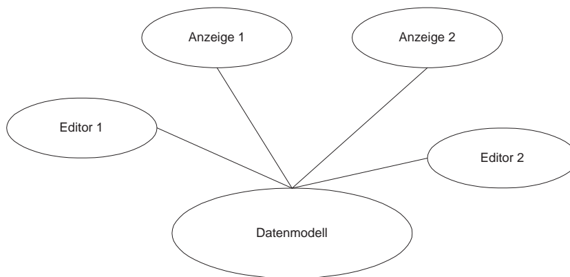
Abbildung 5.4.: Model-View-Mechanismus
