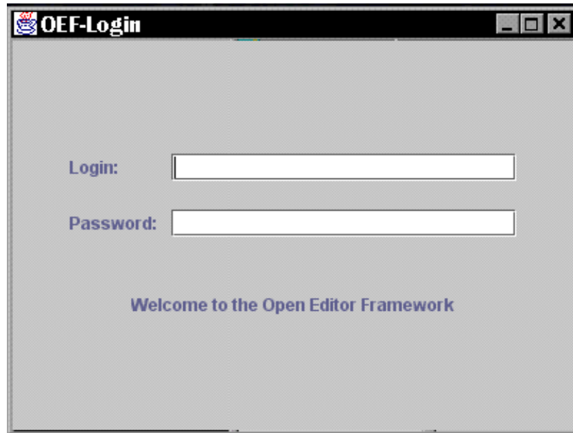
Abbildung 3.1.: Login Dialog
