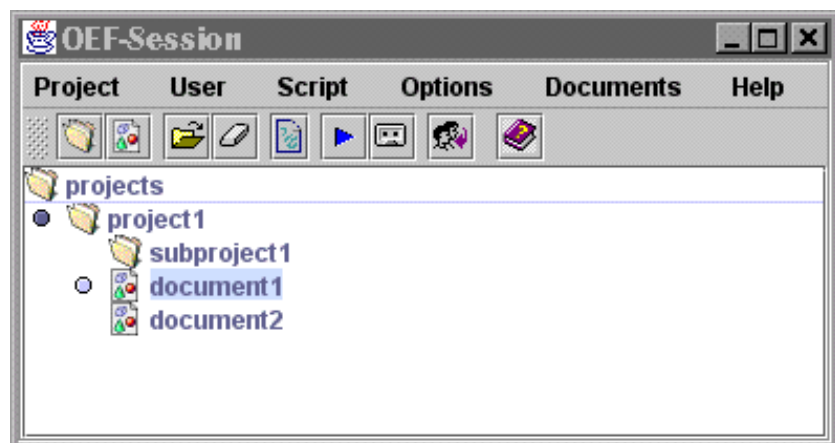
Abbildung 3.2.: Projektmanager
