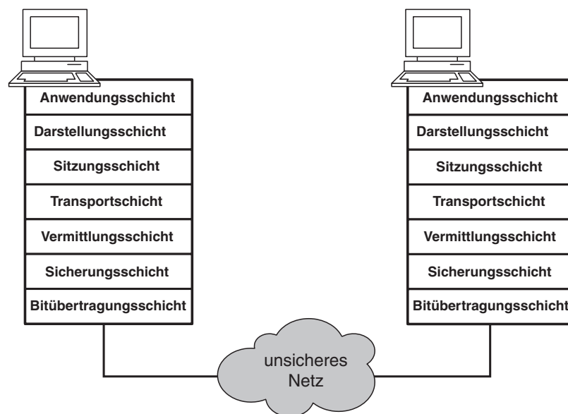
Abbildung 2: Das OSI-Referenzmodell
