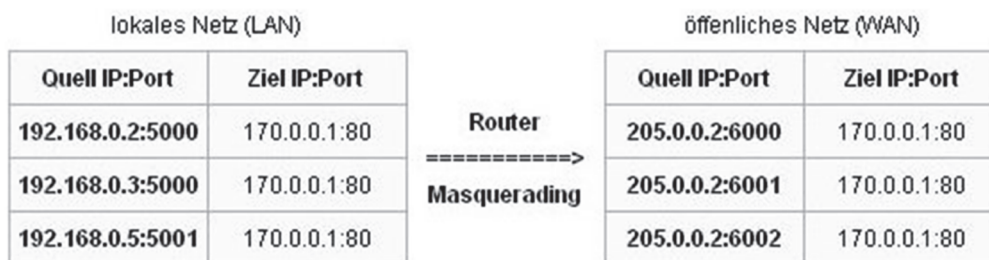
Abbildung 22: Masquerading
