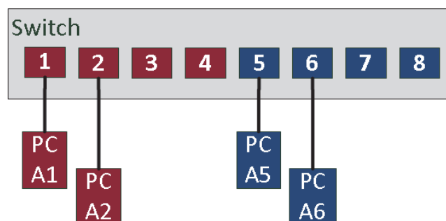
Abbildung 23: VLAN-Switch mit zwei VLANs
