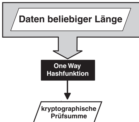
Abbildung 28: One-Way-Hashfunktion
