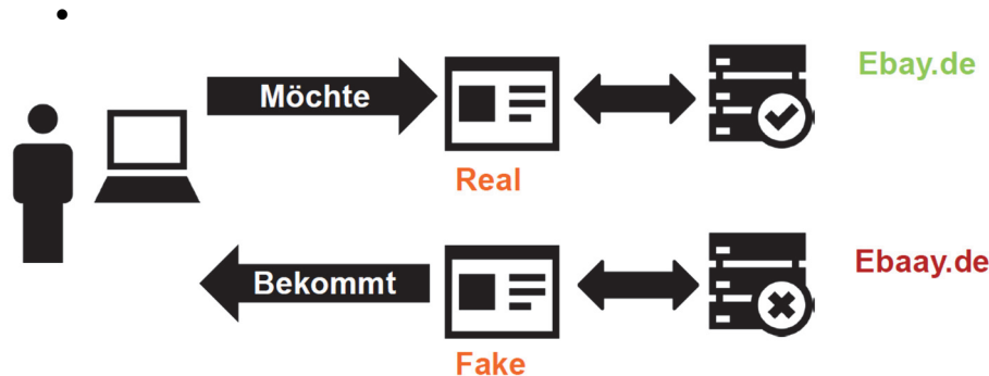
Abbildung 33: Phishing-Angriff
