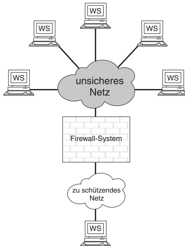
Abbildung 21: Firewall-System
