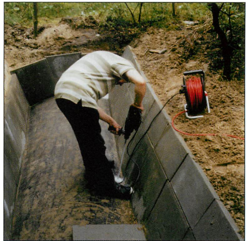
Abb. 15. Winterquartier Nr. 11: Bleckede Tonnengang. Das Regenfangbecken wurde direkt im Zenitbereich über dem Gang gebaut.
