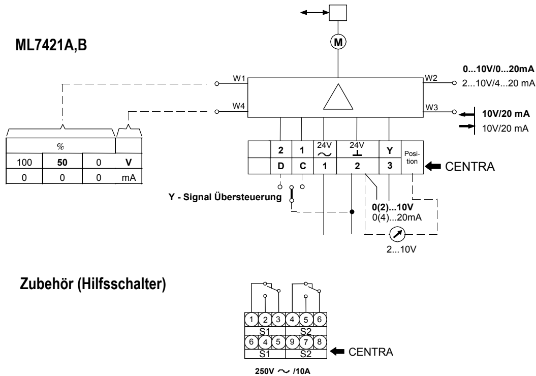
Abb. 3 Anschluss
