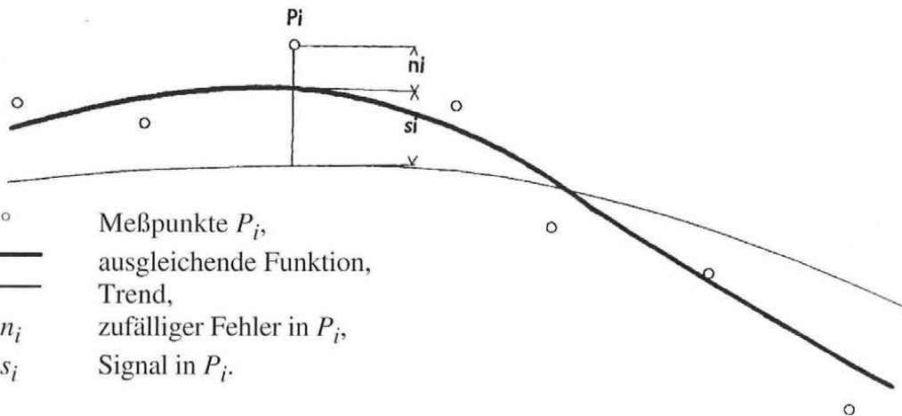
Abb. 3.5: Prinzip der Kollokation
