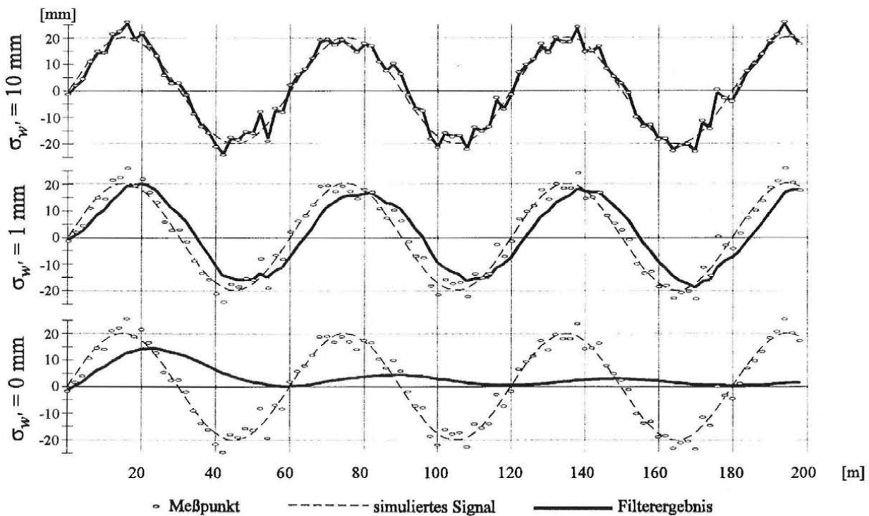
Abb. 4.9: Filterergebnisse bei einem Systemmodell 1. Ordnung und unterschiedlichen Werten für die Standardabweichung des Systemrauschens \sigma_{w'}
