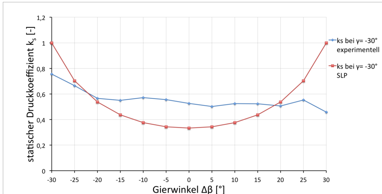
Abbildung 6.18: statischer Druckkoeffizient k_s für den Nickwinkel von \Delta\gamma = -30^\circ bei der SVUSS/3 Kobrasonde
