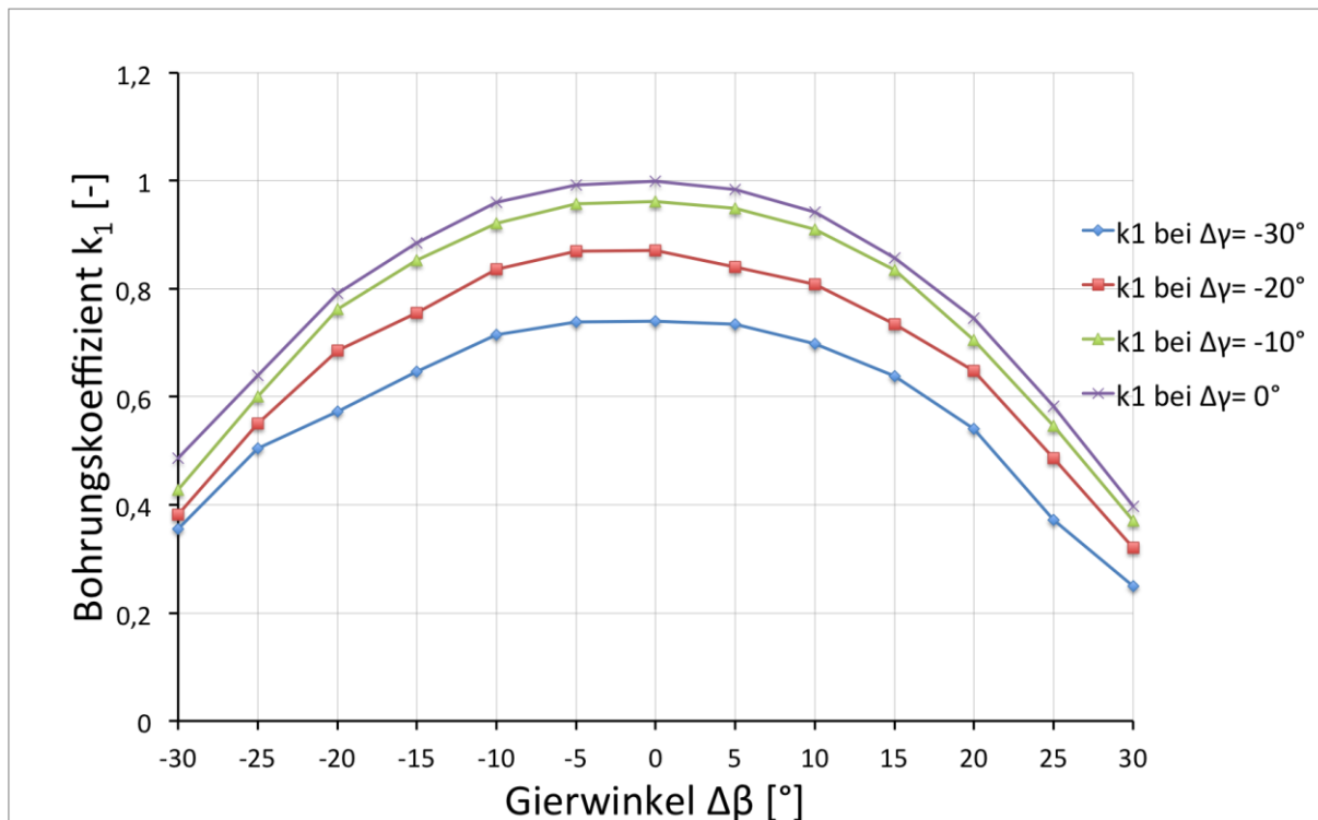
Abbildung 6.40: Bohrungskoeffizient k_1 für den Nickwinkelbereich von \Delta\gamma = -30^\circ bis 0^\circ bei der AVA Zylindersonde Nr. 43
