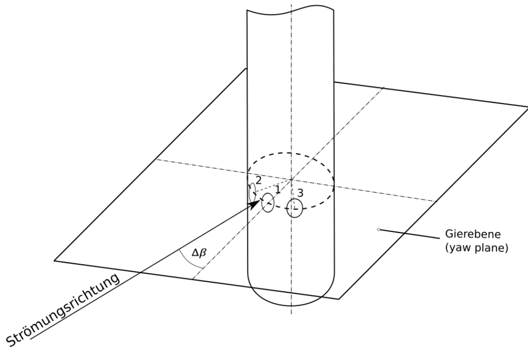
Abbildung 2.1: zylindrische Dreilochsonde mit Anströmwinkel \Delta\beta
