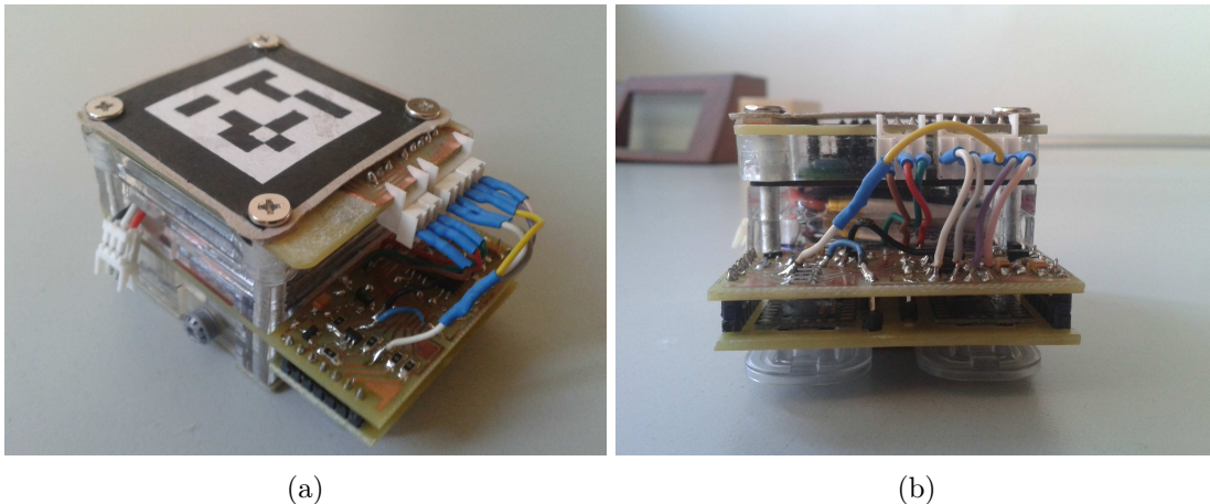
Abbildung 20: Finaler Prototyp auf ACTO: (a) von oben mit Marker, (b) von vorne
