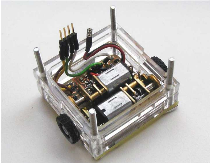
Abbildung 5: ACTO-Motoreinheit [3]
