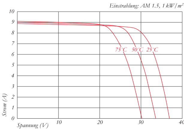
Strom-Spannungs-Kennlinie bei verschiedenen Zelltemperaturen
