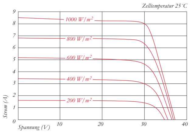
Strom-Spannungs-Kennlinie bei verschiedener Einstrahlung
