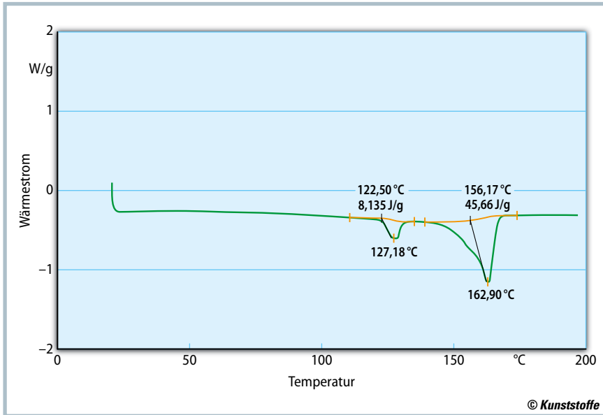
Bild 1. DSC-Analyse der Regranulats PP 580S (2. Aufheizkurve)
