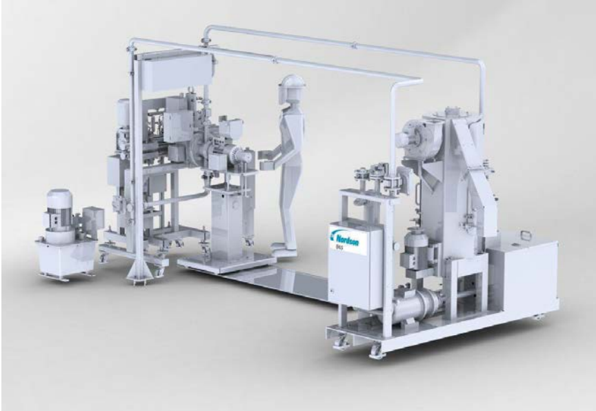
Bild 4. Modell einer Anlage für Unterwassergranulierung
