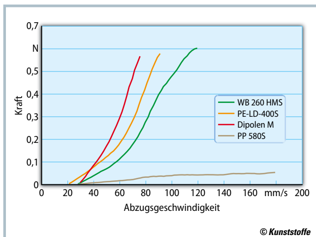
Bild 2. Vergleich der Schmelzfestigkeiten von PP WB 260 HMS, Regranulat Dipolen M, PE-LD-400S und Regranulat PP 580S bei 160°C
