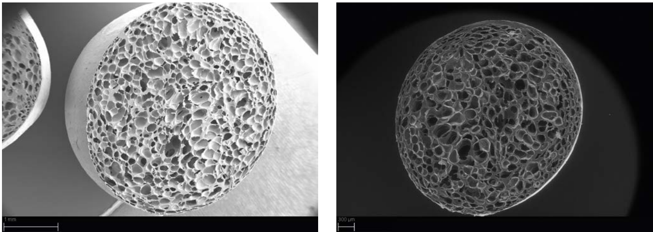
Bild 5. REM-Aufnahme einer geschäumten Perle von PE-LD-400S/WB 260 (links) und von Dipolen M/WB 260 (rechts)
