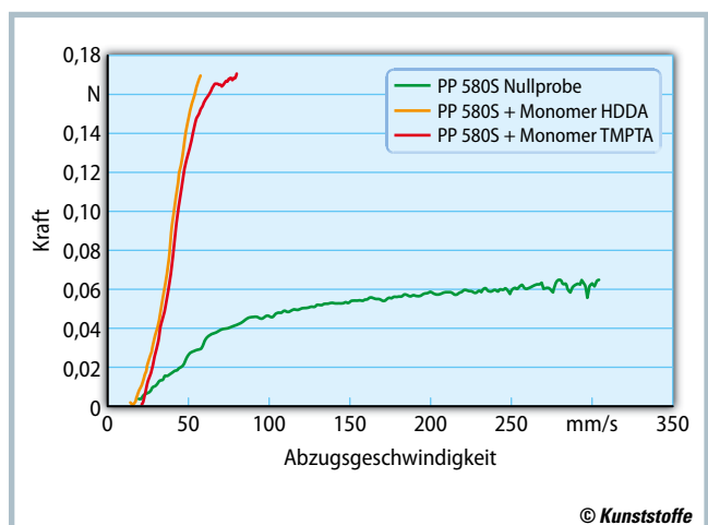
Bild 3. Vergleich der Schmelzfestigkeiten einer Standardprobe des Regranulats PP 580S mit zwei unterschiedlich modifizierten Proben bei 180°C
