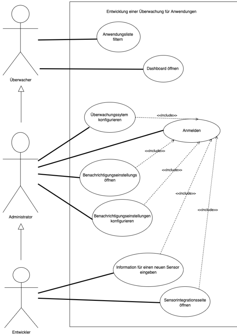
Abbildung 3: Use-case Diagramm
