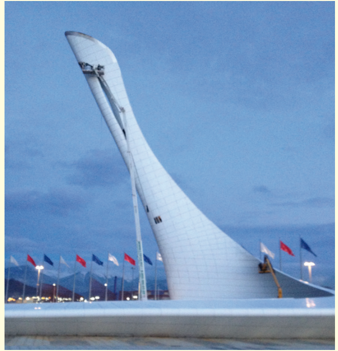
Bild 3. Nahezu fertiggestellte Struktur der olympischen Fackel im Dezember 2013, Durchführung der Schwingungsmessungen vor Ort
