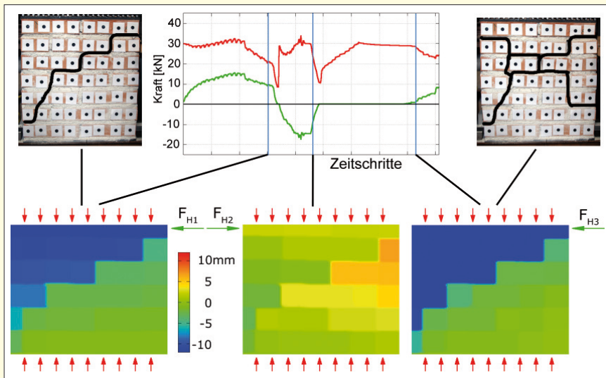
Bild 5: Ergebnisse der Mauerwerksversuche mit Kalkmörtel
