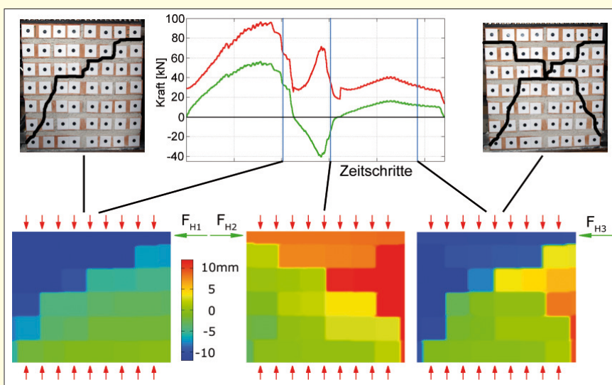
Bild 6: Ergebnisse der Mauerwerksversuche mit Mörtel M10
