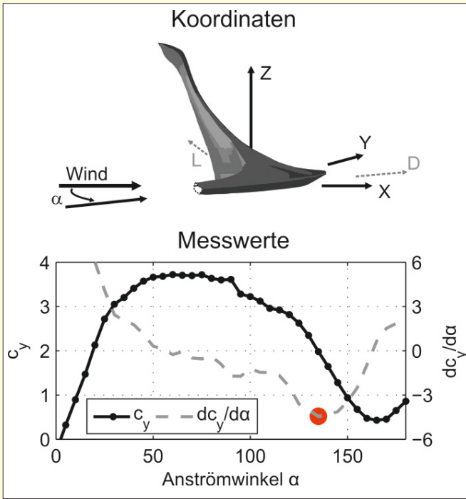
Bild 2 Koordinatendefinition und gemessener Verlauf des Quertriebsbeiwertes c_y sowie Derivatium dc_y/d\alpha
