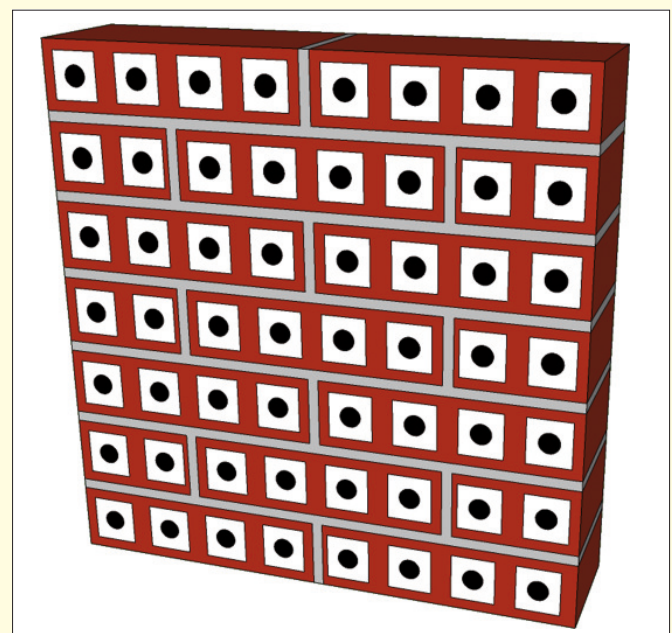
Bild 2: Positionen der 56 Messpunkte für die Videoextensometermessung
