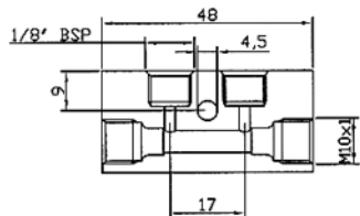
2 Auslässe Teile-Nummer: 3071302
