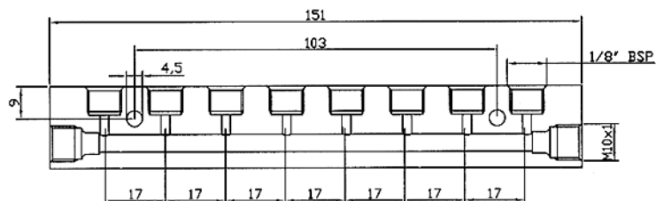
8 Auslässe Teile-Nummer: 3071308
