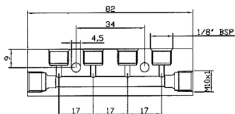
4 Auslässe Teile-Nummer: 3071304
