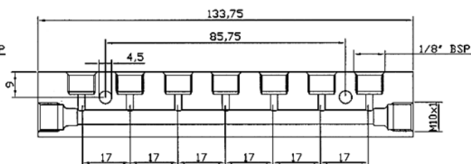
7 Auslässe Teile-Nummer: 3071307
