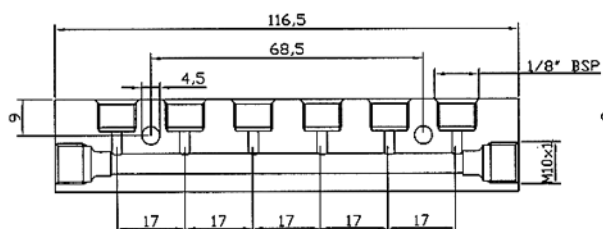
6 Auslässe Teile-Nummer: 3071306
