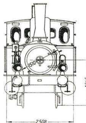
Vorderansicht
