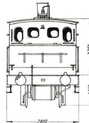
Rückansicht
