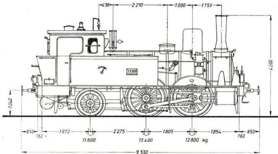
Langsicht
