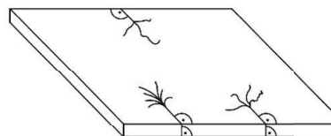
Thermischer Randbruch
