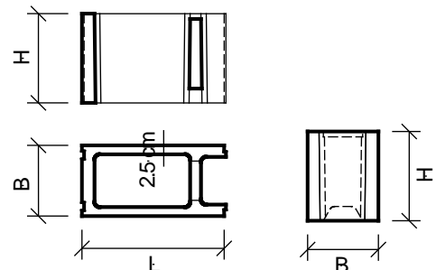
Bild 6: SCHALIT Endstein
