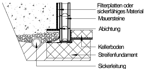
Bild 18 Entwässerung
