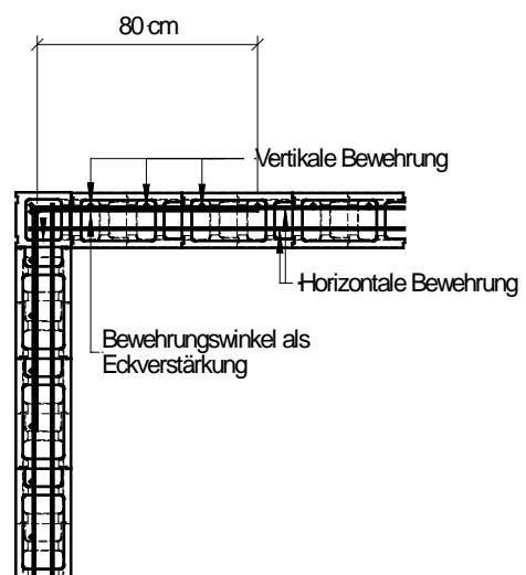
Bild 14: Eckausbildung
