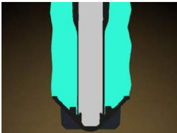
Verpresster Pfahlschuh, Verpresskörper aus Zementmörtel
