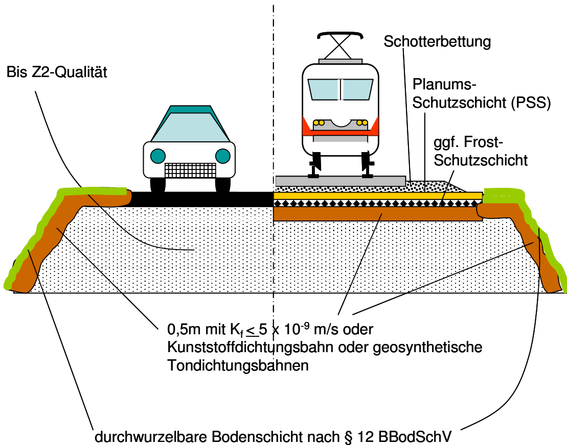
Abbildung 5-8: Kernbauweise als Z2-Einbaukonfiguration
