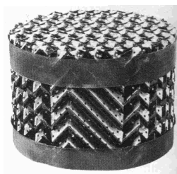
Abb. 9: Füllkörper sowie eine strukturierte Packung und Aufbau einer Packungskolonne
