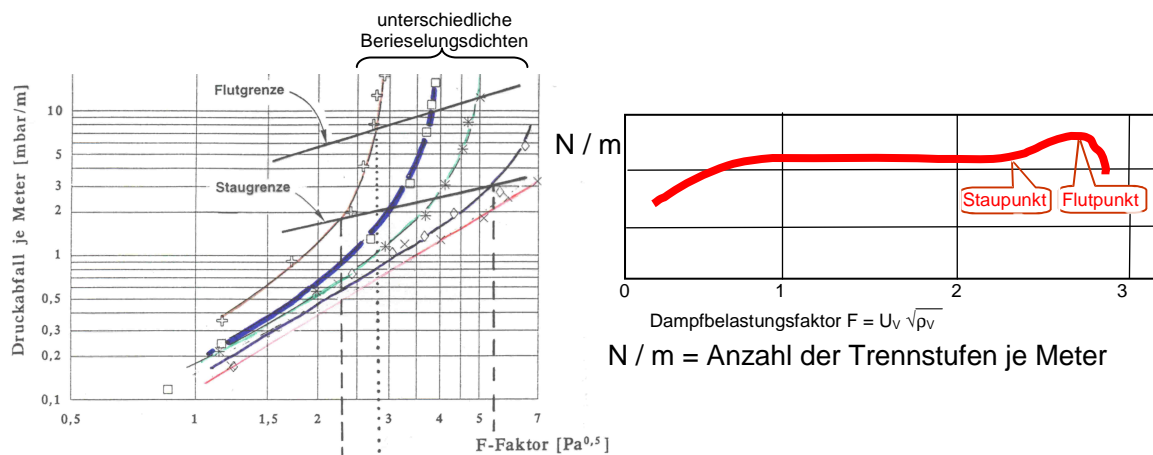
Abb. 10: spezifischer Druckverlust und Anzahl der theoretischen Trennstufen/m (NTU/m) als Funktion des F-Faktors (F = Dampfgeschwindigkeit im freien Querschnitt * \sqrt{\text{Dampfdichte}} )
