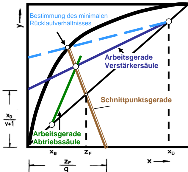
Abb. 6: Gleichgewichtsdiagramm mit Verstärkungs-, Abtriebs- und Schnittpunktgeraden
