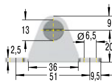
MA5 Lagerschuh
