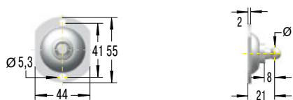
PG5 Rundbeslag
