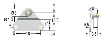
OG5 Seitenbeslag
