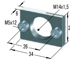
RF14 Rechteckflansch
