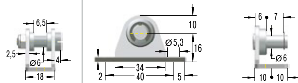
NA5 Winkelbeslag
