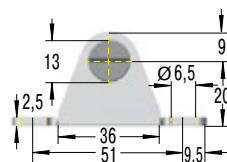
MA10-V4A Lagerschuh
