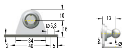
NG5 Winkelbeslag
