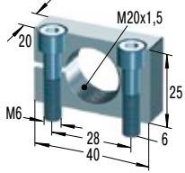
MB20 Klemmflansch
