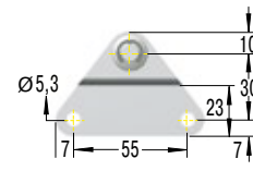
OG8-V4A Seitenbeschlag
