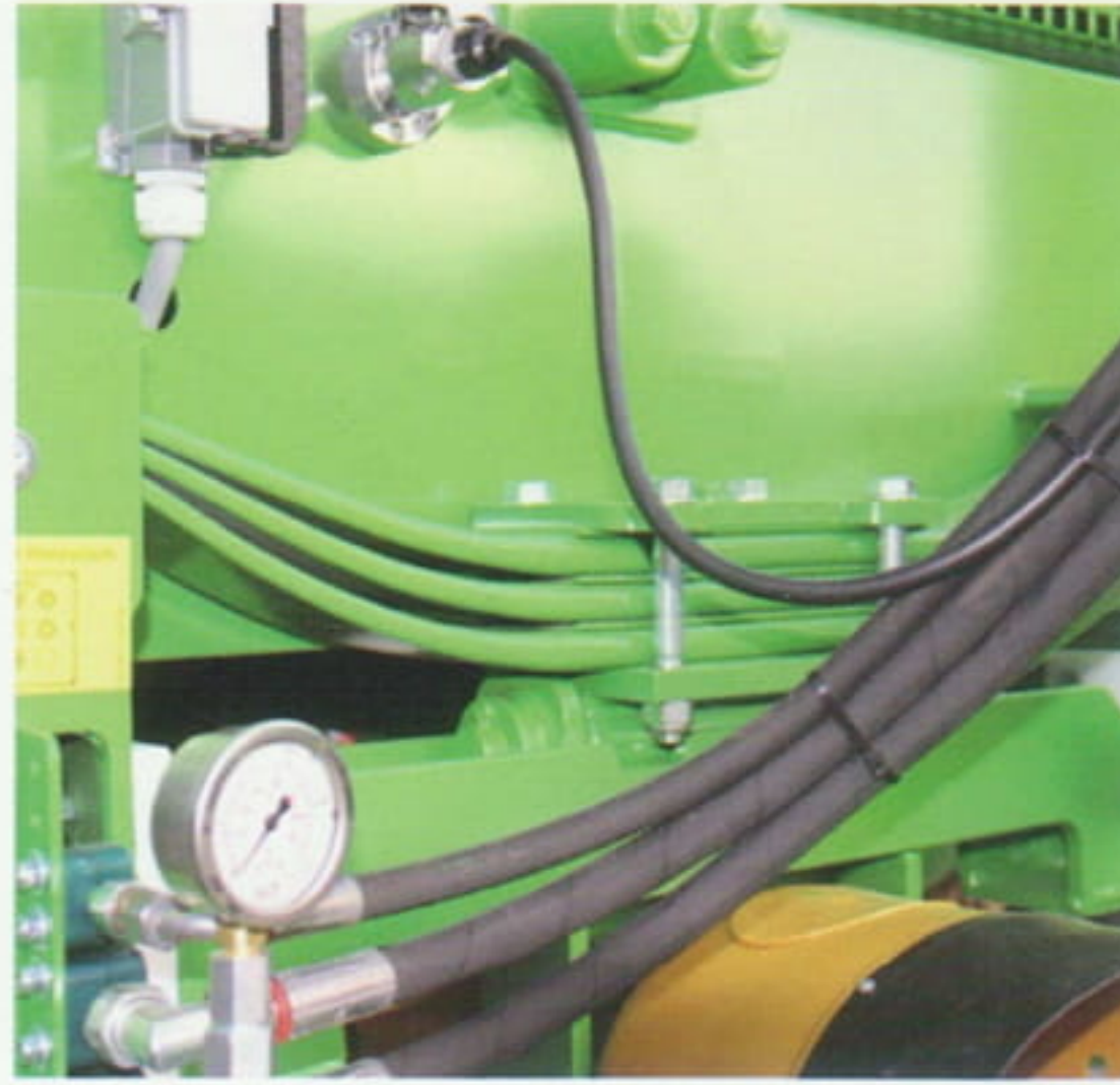
Zugdeichsel, mechanisch gefedert mit Oben-/Untenanhängung.
