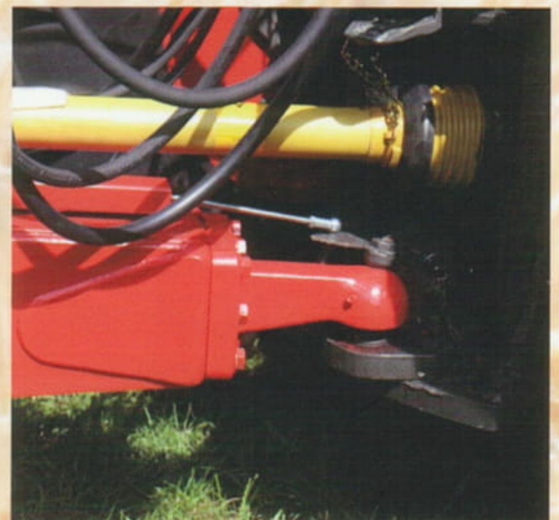
Ansteuerung der Zwangslenkung durch Bowdenzug.
