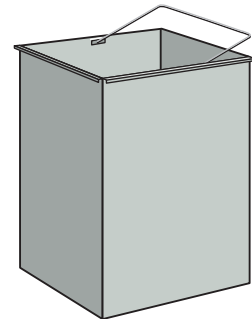
Innenbehälter Modell 16/BI-AU – dichtgeschweißt – mit Tragebügel 70 l Fassungsvermögen – dieser Innenbehälter wird bei Behältern mit Ausschnitt einge- setzt, passend für 16/BF und 16/BF-0
