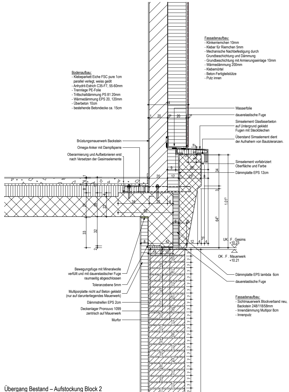
Übergang Bestand – Aufstockung Block 2
