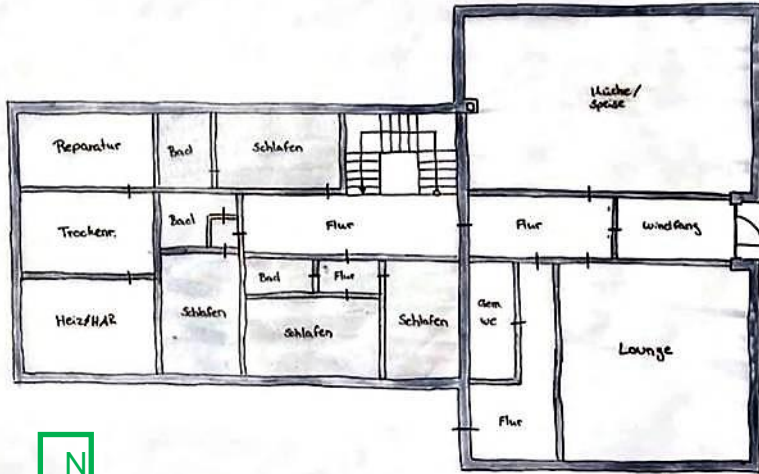
Grundriss EG
