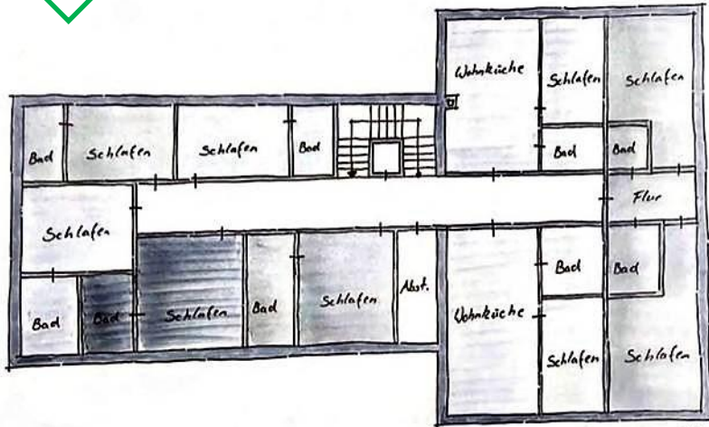
GRUNDRISS OG
