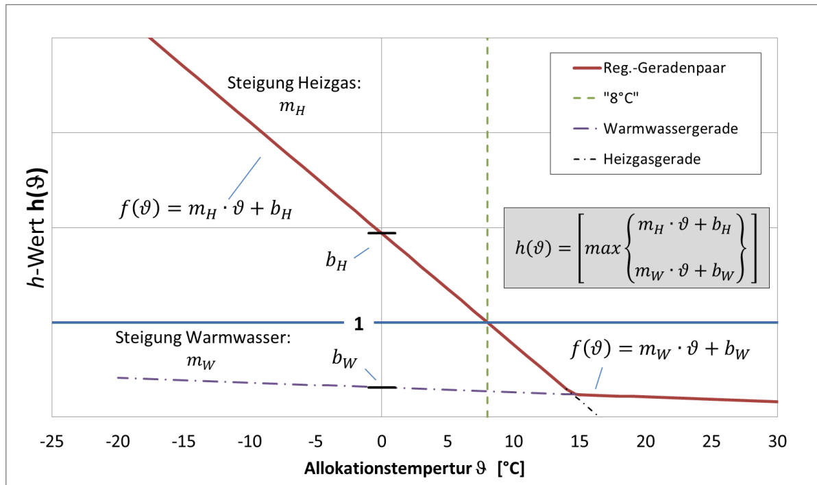
Abbildung 33 Wirkungsweise des Regressionsgeradenpaar
