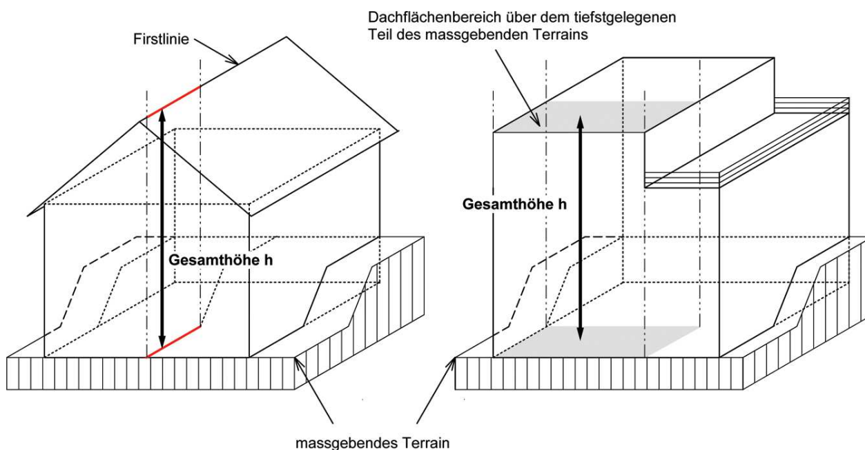
Figur 5.1 Gesamthöhe
