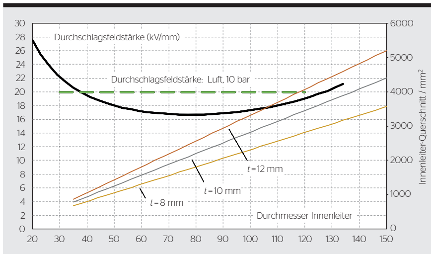
Bild 3 Einfluss des Innenleiter-Durchmessers auf die maximale Feldstärke bei Aussenleiter-Durchmesser von 212 mm und 650 kV.
