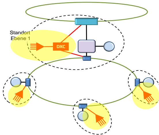
Abbildung 6-2: Layer 1 Integration elektrisch (NG-SDH) – Netzebene 0-1
