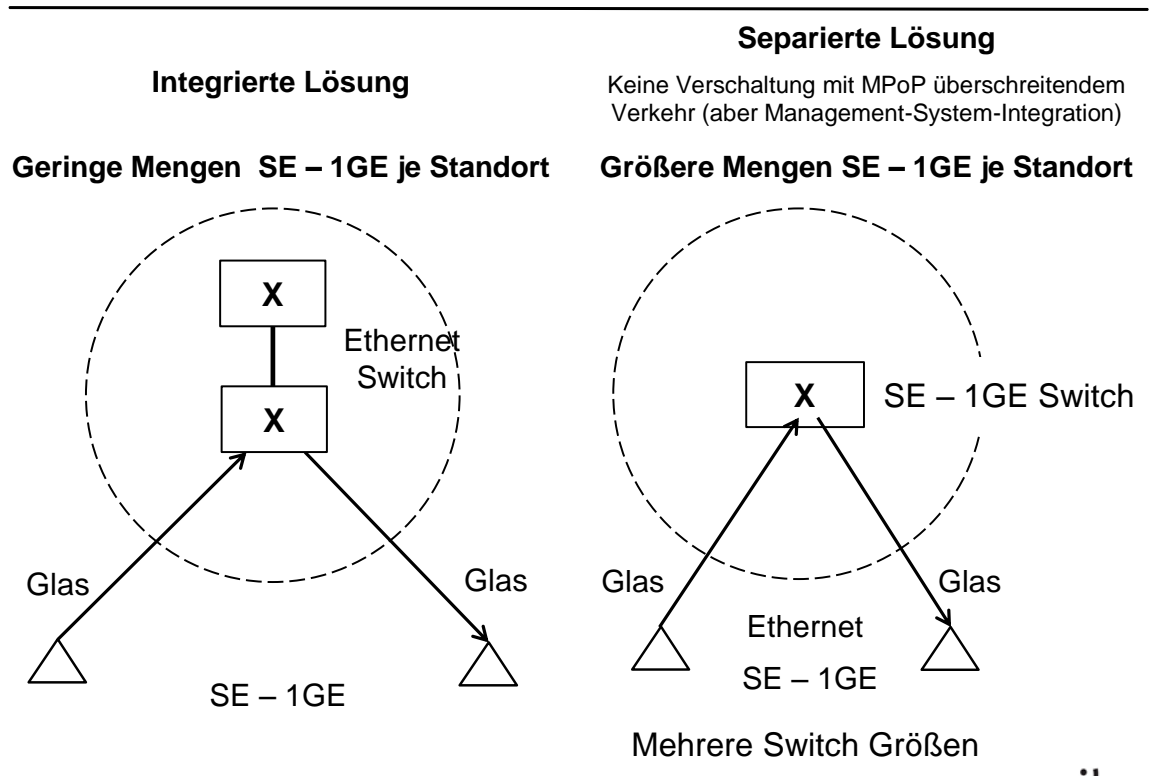
Abbildung 6-12: Standortinterne Verbindungsnachfragen Layer 2 von SE bis zu GE
