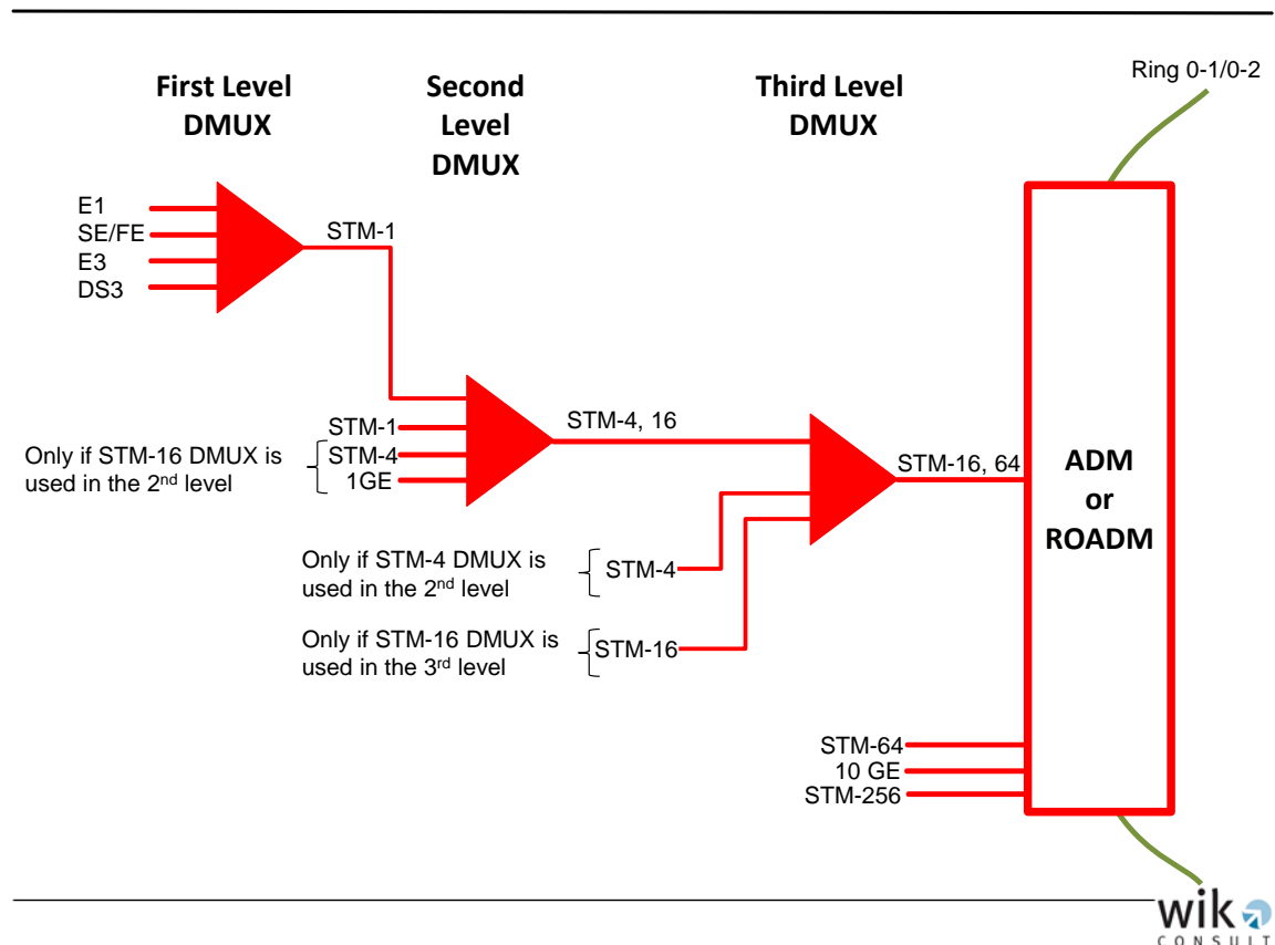
Abbildung 6-1: Kaskadierung der Anschlussnachfrage
