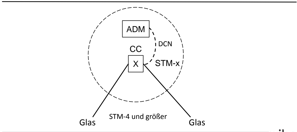
Abbildung 6-9: Fall 3: Größere Mengen von großen standortinternen Verbindungen (STM-4 und größer)
