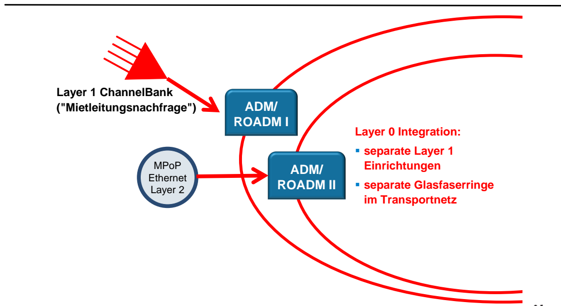
Abbildung 6-14: Layer 0 Integration der spezifischen Layer 1 Verbindungsnachfragen
