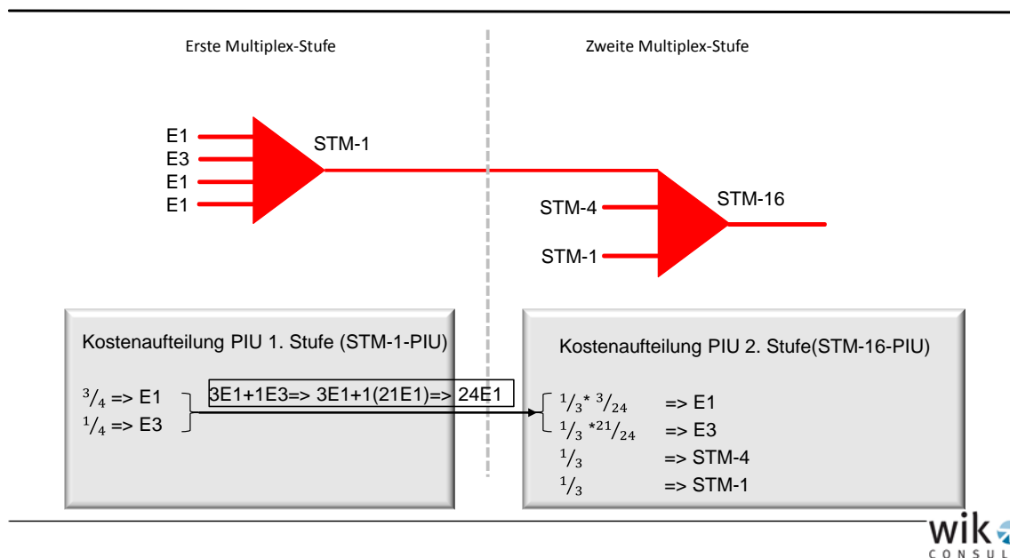
Abbildung 8-4: Kostenzurechnung anschließendes und aggregierendes Equipment am MPoP am Beispiel von SDH
