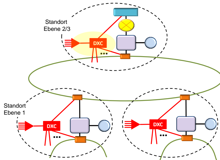
Abbildung 6-4: Layer 1 Integration optisch (DWDM) – Netzebene 1-2/3
