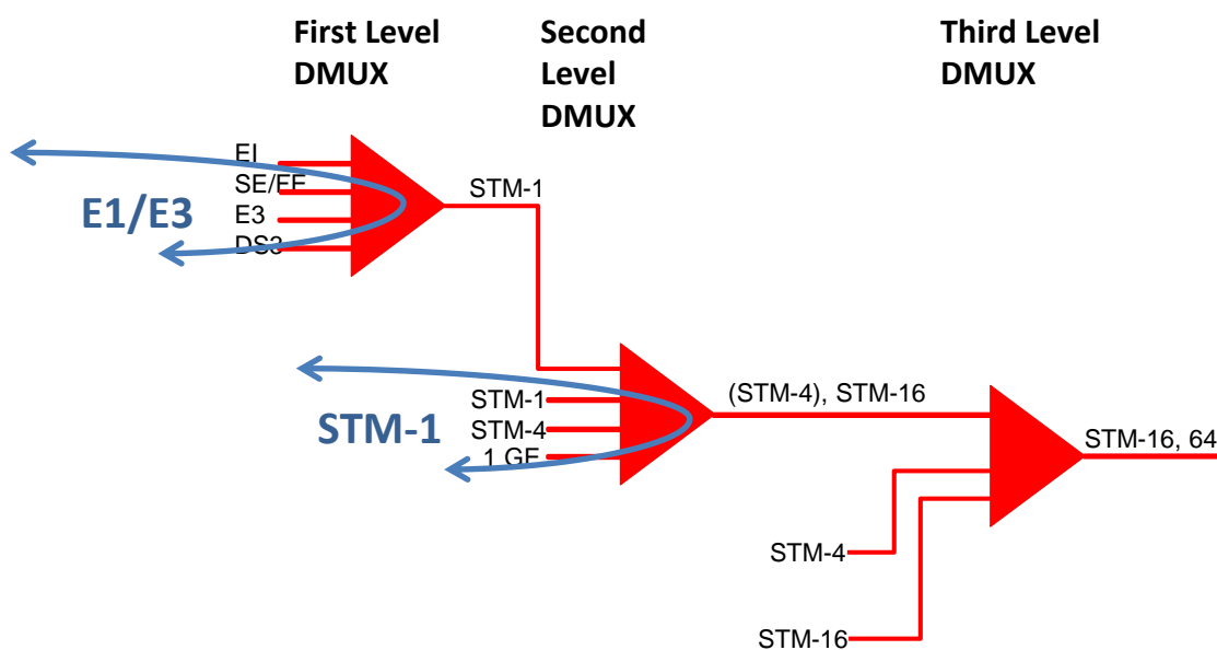
Abbildung 6-6: Fall 1: Integrierte E1 Realisierung für geringe Anzahl interner Verbindungsnachfragen
