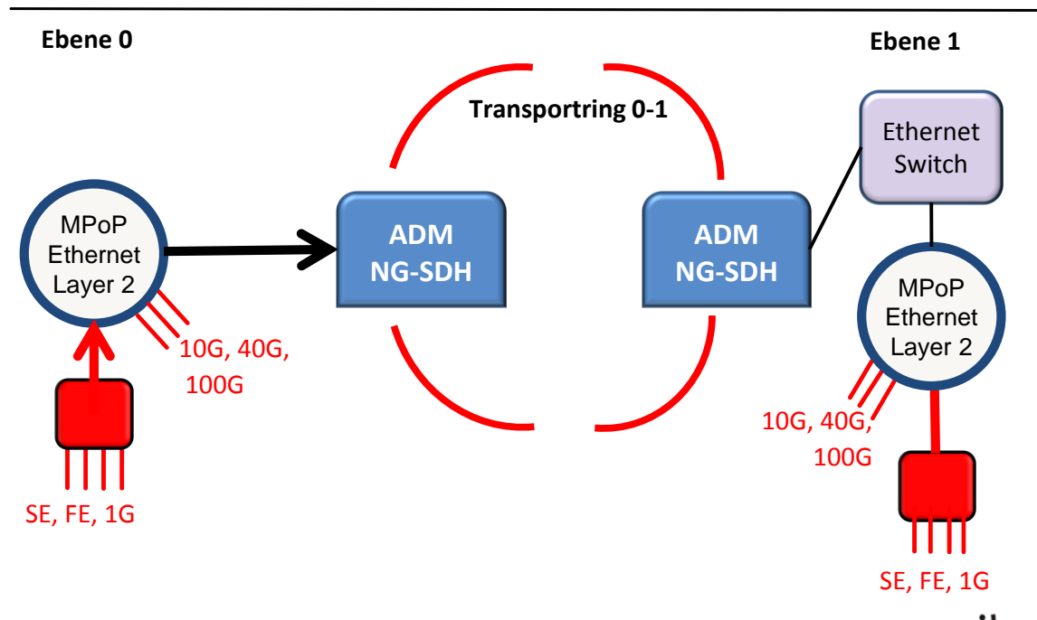
Abbildung 6-10: Anschluss und Aggregation von Layer 2 Kapazitätsnachfragen
