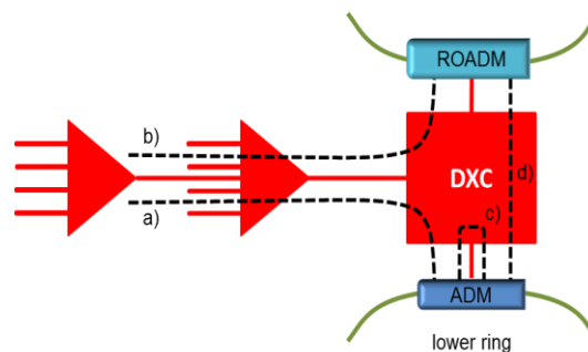
Abbildung 6-3: Steuerung der Verbindungsnachfragen im DXC
