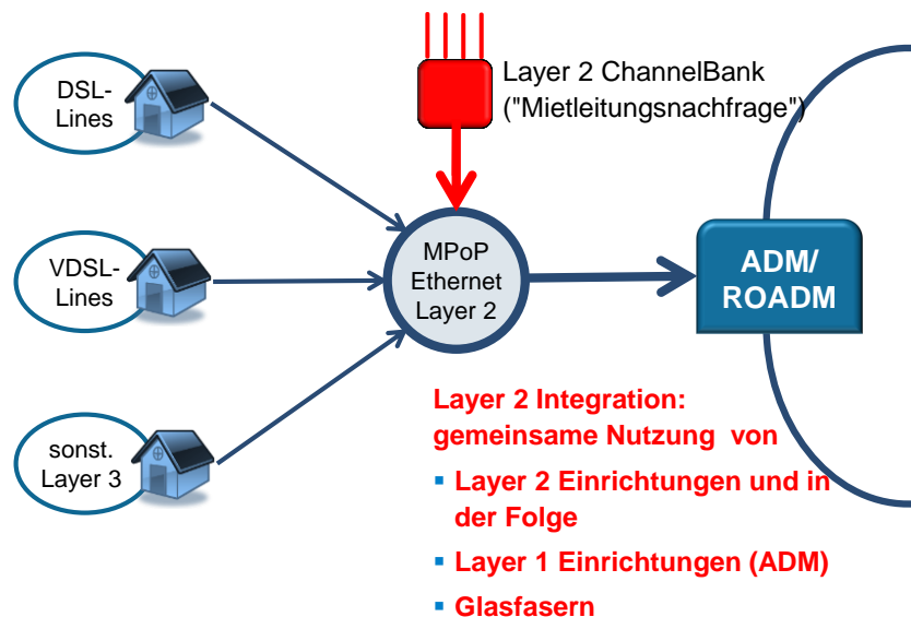
Abbildung 4-3: Layer 2 Integration der spezifischen Layer 2 Kapazitätsnachfragen
