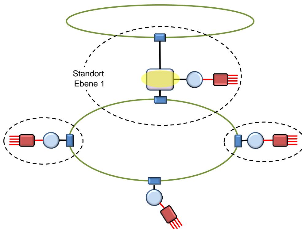
Abbildung 6-11: Steuerung der Ethernet Mietleitungen durch hierarchisch übergeordneten Ethernet-Switch des Breitbandnetzes
