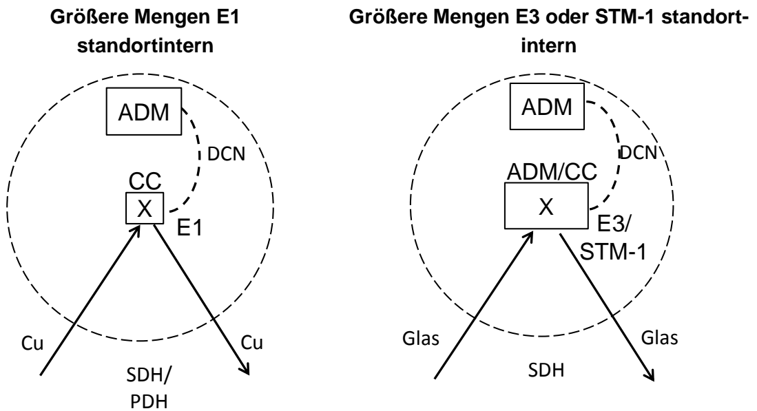
Abbildung 6-8: Fall 3: Größere Mengen von kleinen und mittleren Größen einer standortinternen Verbindungsnachfrage (E1, E3, STM-1)
