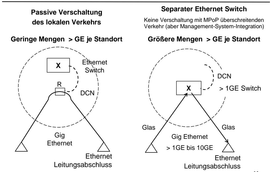
Abbildung 6-13: Standortinterne Verbindungsnachfragen Layer 2 von mehr als 1GE
